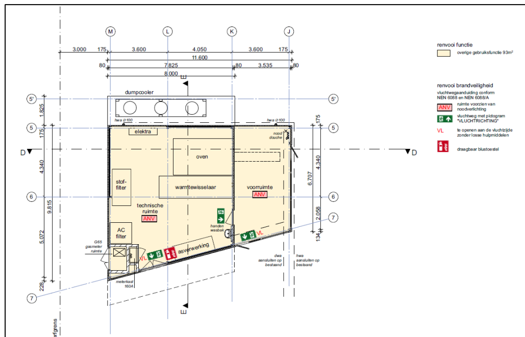
Ontwerp, Technisch crematorium Gorinchem
