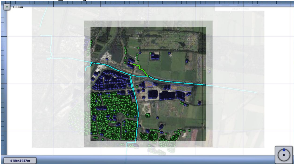
Figuur 4.4 Kilometer leiding behorende bij de maximale overschrijding van de FN-curve voor 5365_leiding-W-528-15-deel-1 van N.V. Nederlandse Gasunie
