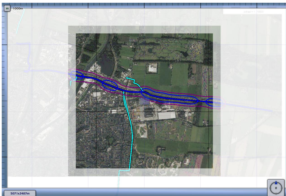
3.1 Figuur 3.1 Plaatsgebonden risico voor 5365_leiding-W-528-01-deel-1 van N.V. Nederlandse Gasunie
