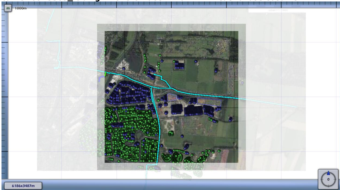
Figuur 4.3 Kilometer leiding behorende bij de maximale overschrijding van de FN-curve voor 5365_leiding-W-528-07-deel-1 van N.V. Nederlandse Gasunie
