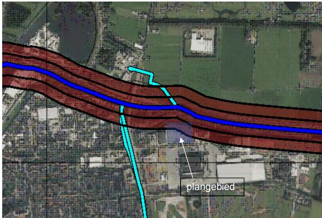
Figuur 2.1: Uitsnede CAROLA invloedsgebied buisleiding
