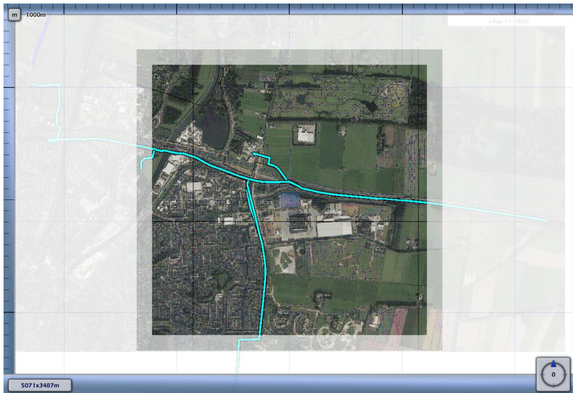
3.3 Figuur 3.3 Plaatsgebonden risico voor 5365_leiding-W-528-07-deel-1 van N.V. Nederlandse Gasunie
