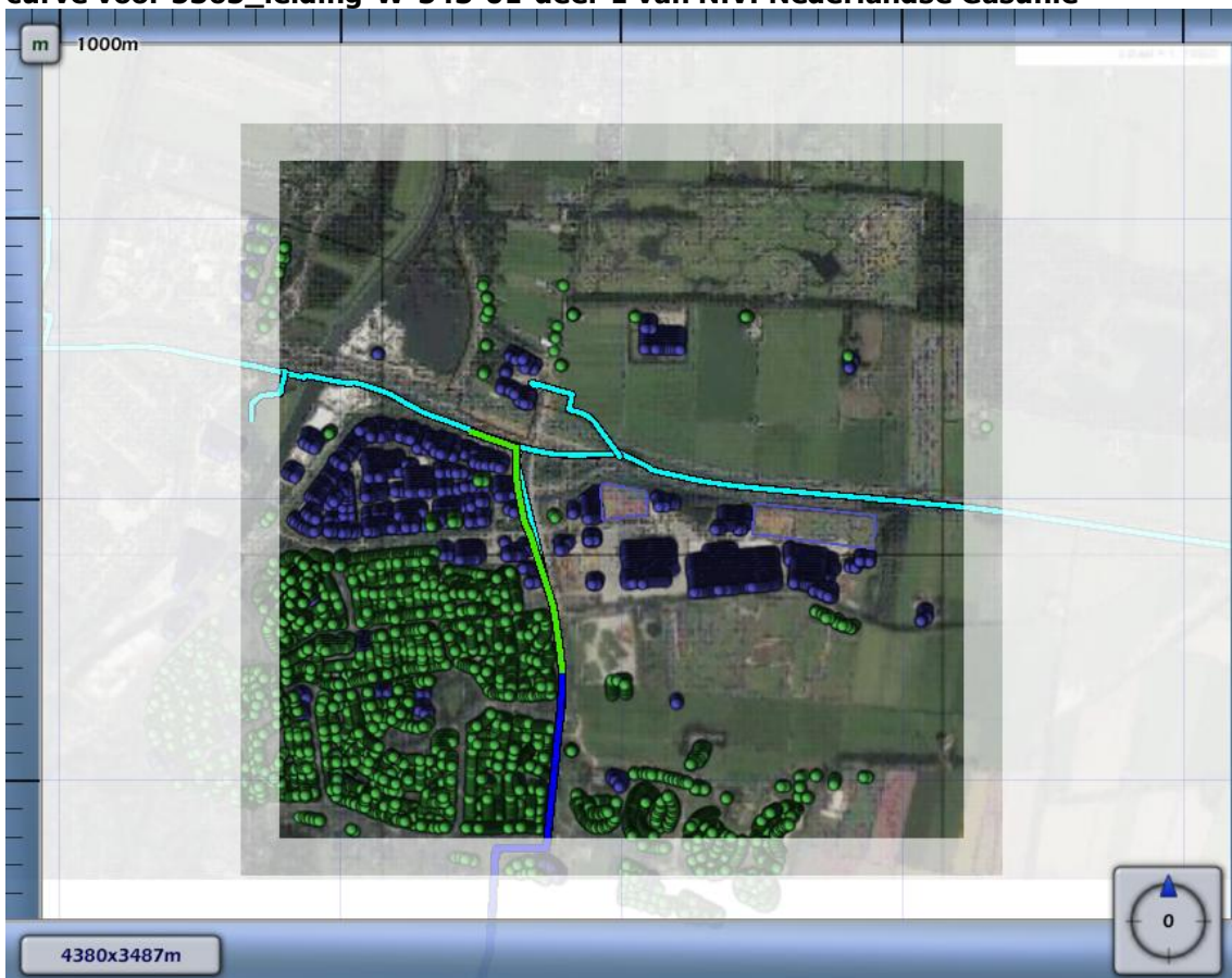
Figuur 4.5 Kilometer leiding behorende bij de maximale overschrijding van de FN-curve voor 5365_leiding-W-543-01-deel-1 van N.V. Nederlandse Gasunie
