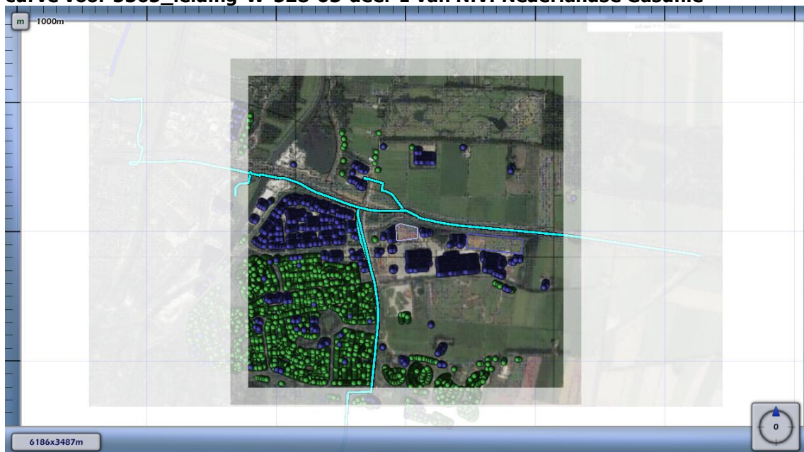
Figuur 4.2 Kilometer leiding behorende bij de maximale overschrijding van de FN-curve voor 5365_leiding-W-528-03-deel-1 van N.V. Nederlandse Gasunie
