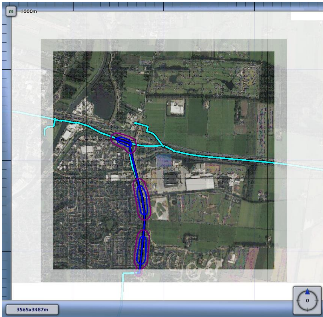
3.6 Figuur 3.6 Plaatsgebonden risico voor 5365_leiding-W-543-02-deel-1 van N.V. Nederlandse Gasunie
