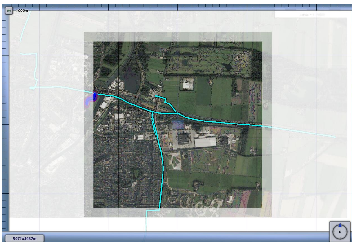
3.3 Figuur 3.3 Plaatsgebonden risico voor 5365_leiding-W-528-07-deel-1 van N.V. Nederlandse Gasunie
