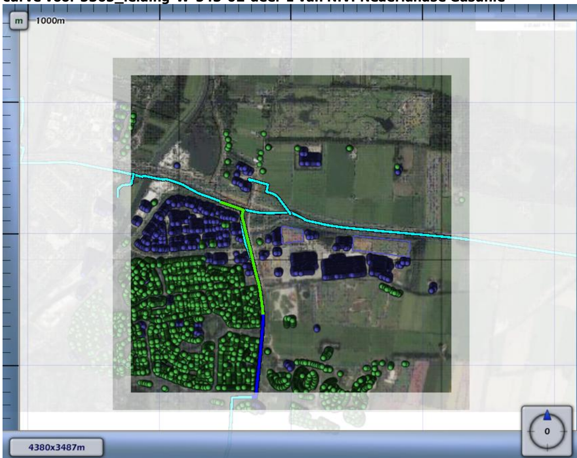
Figuur 4.6 Kilometer leiding behorende bij de maximale overschrijding van de FN-curve voor 5365_leiding-W-543-02-deel-1 van N.V. Nederlandse Gasunie
