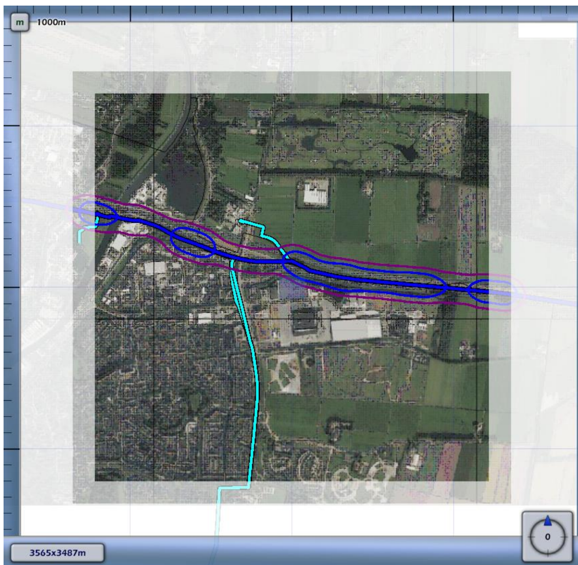
3.1 Figuur 3.1 Plaatsgebonden risico voor 5365_leiding-W-528-01-deel-1 van N.V. Nederlandse Gasunie
