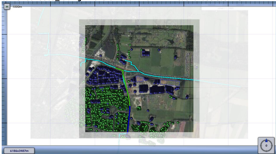
Figuur 4.6 Kilometer leiding behorende bij de maximale overschrijding van de FN-curve voor 5365_leiding-W-543-02-deel-1 van N.V. Nederlandse Gasunie
