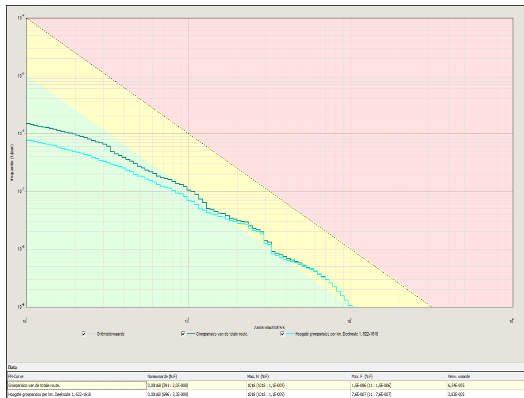
Grafiek 5.2: fN-curve berekend groepsrisico toekomstige situatie
