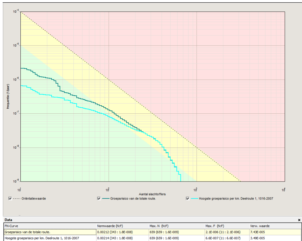
Grafiek 4.1: fN-curve berekend groepsrisico A15 - huidige situatie
