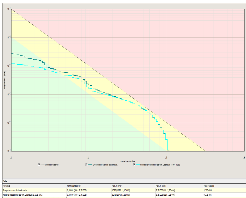
Grafiek 4.2: fN-curve berekend groepsrisico A15 - toekomstige situatie
