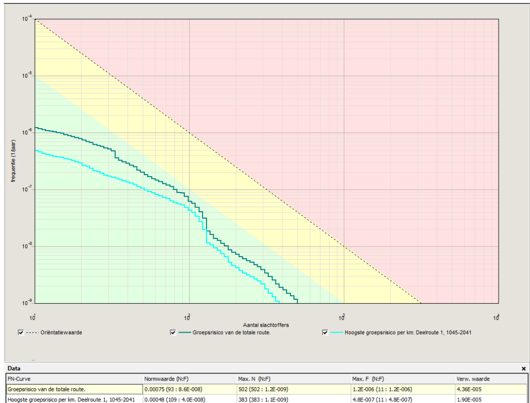
Grafiek 5.1: fN-curve berekend groepsrisico huidige situatie
