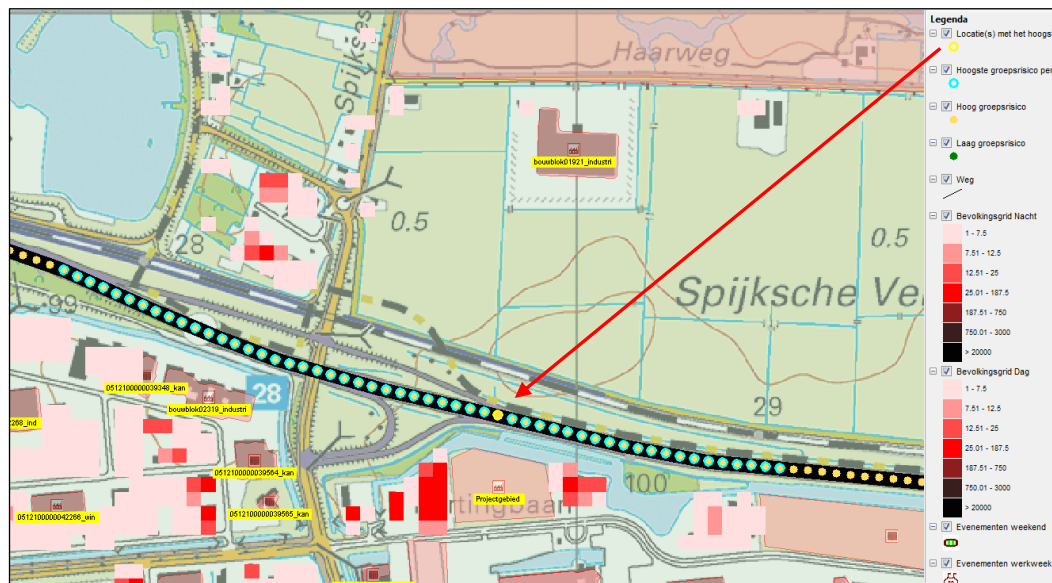
Figuur 4.3: Locatie met hoogste GR weg (A15) - toekomstige situatie
