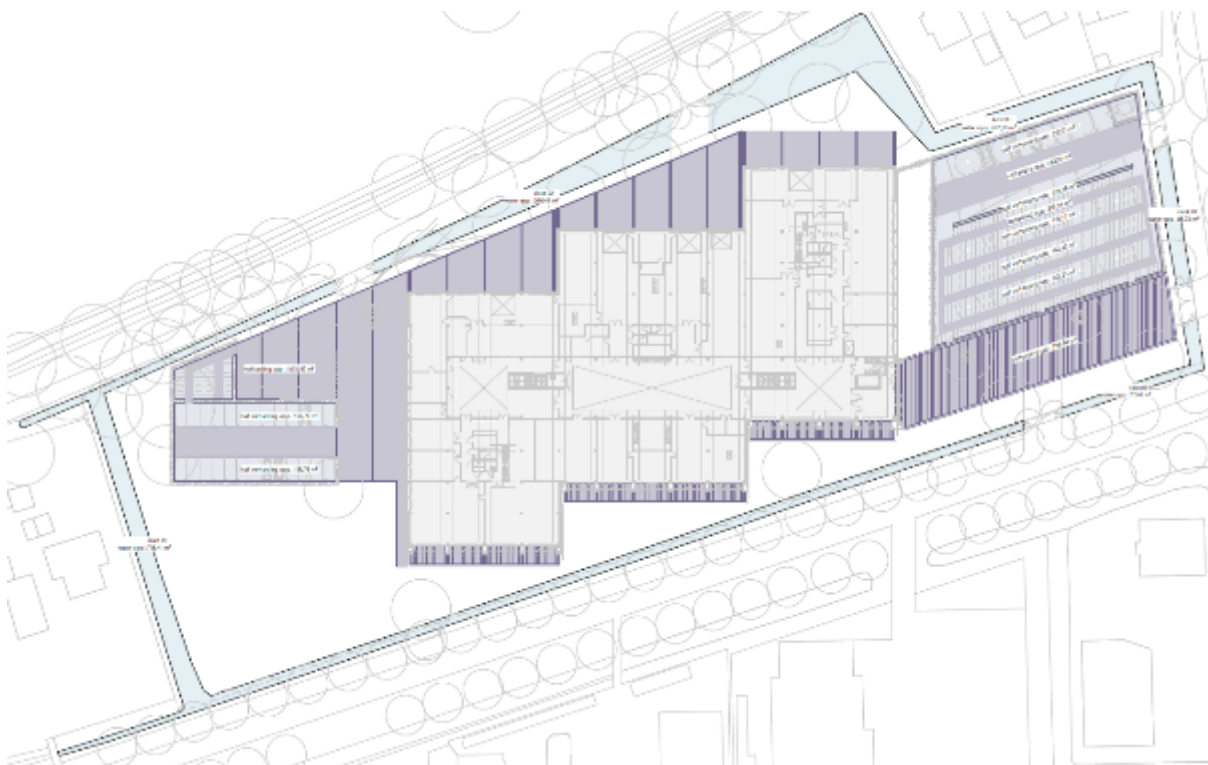
Figuur 5.2: waterhuishoudkundig plan
