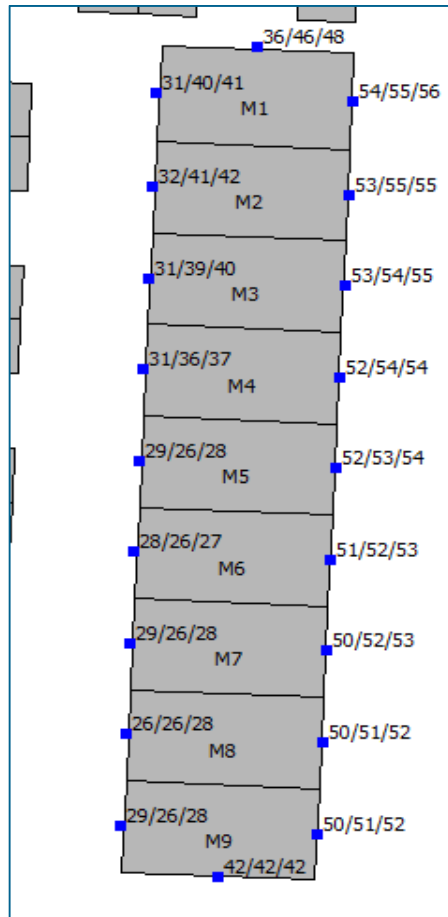
Figuur 4.7 Geluidbelastingen van Cornelis Trompweg op gebouw Midden exclusief ex. Art. 110g Wgh.
