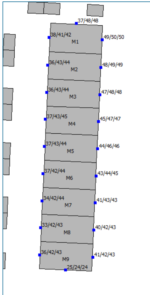
Figuur 4.4 Geluidbelastingen van Van Kinsbergenstraat op gebouw Midden exclusief ex. Art. 110g Wgh.
