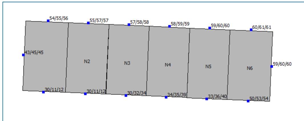
Figuur 4.5 Geluidbelasting van de Cornelis Trompweg op gevels gebouw Noord (excl. Aftrek ex. Artikel 110g Wgh).
