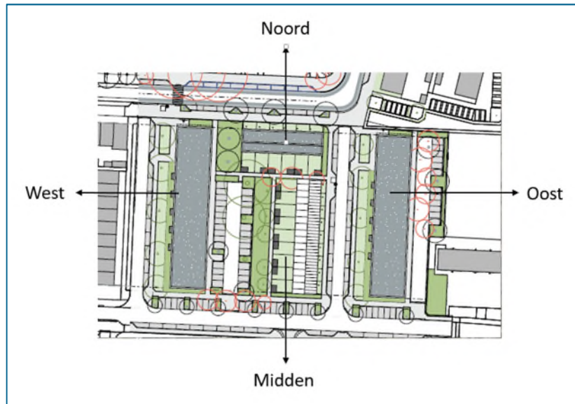
Figuur 3.2 Indeling gebouw namen
