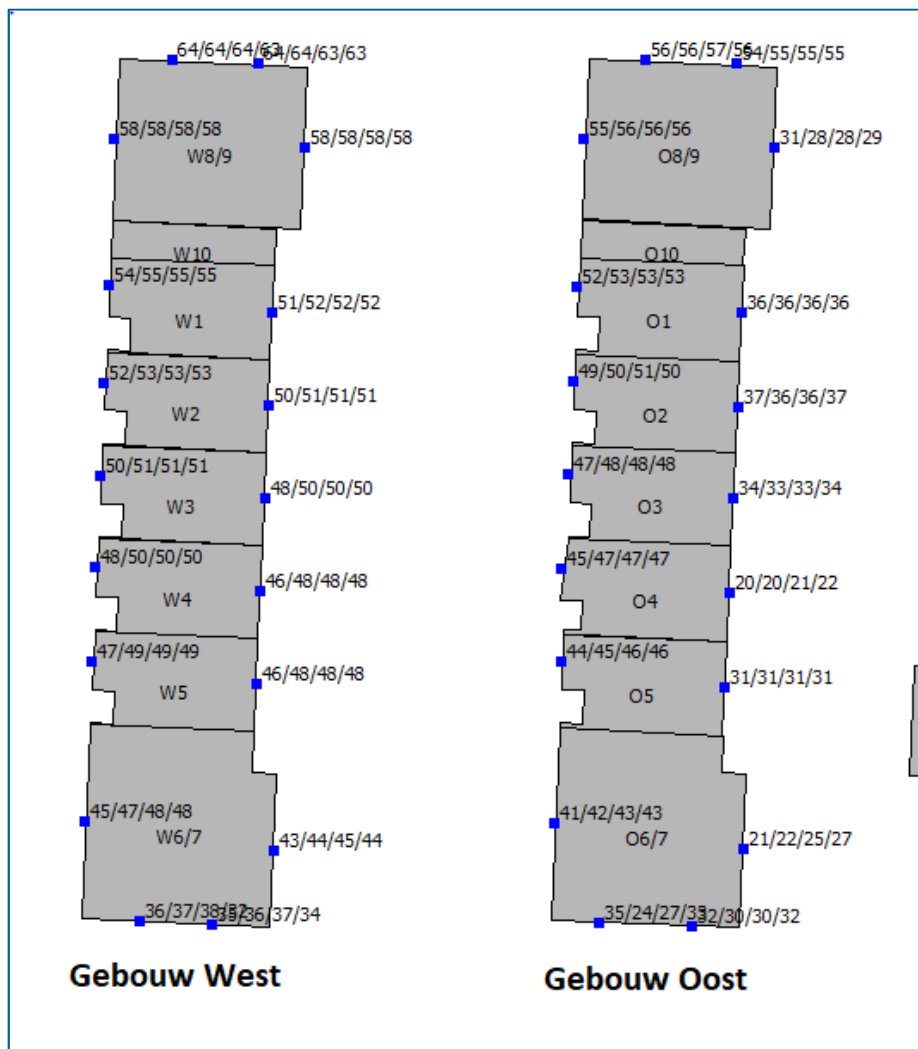
Figuur 4.3 Geluidbelastingen van Van Kinsbergenstraat op gebouwen West en Oost exclusief ex. Art. 110g Wgh.
