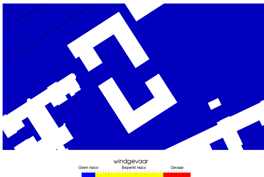
Figuur 4.6: Windgevaar op voetgangersniveau ter plaatse van de nieuwbouw (het Rijn-Schiekanaal tussen de zwarte lijnen)
