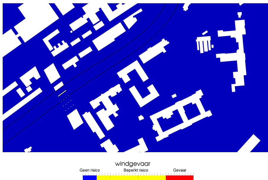
Figuur 4.5: Windgevaar op voetgangersniveau (het Rijn-Schiekanaal tussen de zwarte lijnen)
