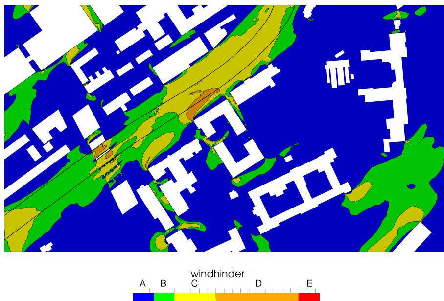
Figuur 4.3: Windhinder op voetgangersniveau (het Rijn-Schiekanaal tussen de zwarte lijnen)
