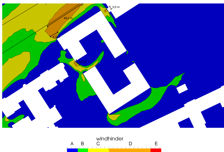
Figuur 4.8: Windhinder op voetgangersniveau ter plaatse van de nieuwbouw, na toevoeging van het trappenhuis aan Kanaalweg 4 (het Rijn-Schiekanaal tussen de zwarte lijnen - in maatvoering de maximale doorlooptegte door windhinderklasse D)
