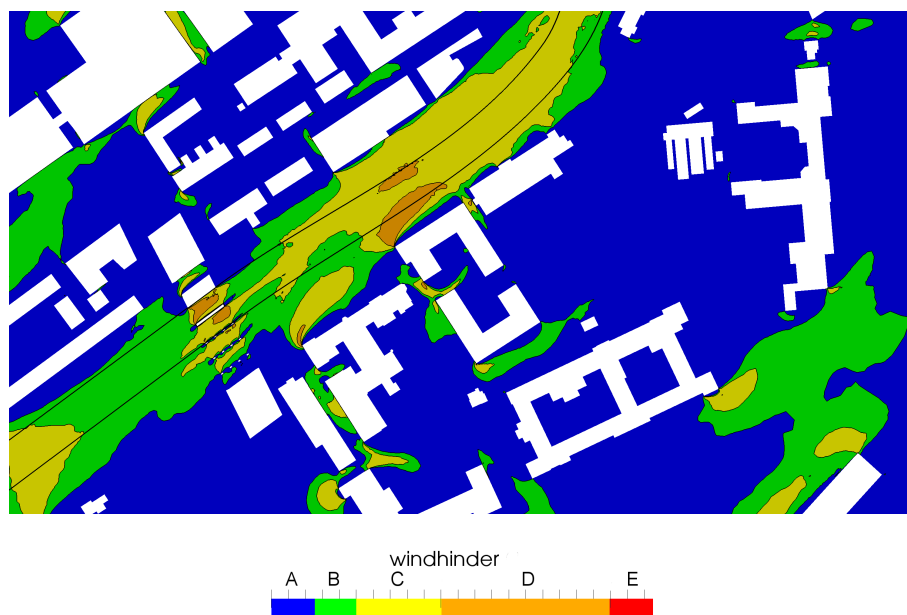
Figuur 4.7: Windhinder op voetgangersniveau, na toevoeging van het trappenhuis aan Kanaalweg 4 (het Rijn-Schiekanaal tussen de zwarte lijnen)
