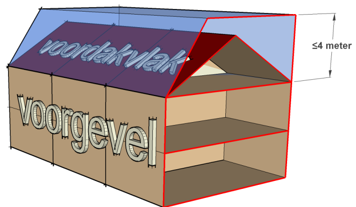
Aanzicht voorzijde "langskap" Kapprofiel B: \leq 55^\circ en \leq 4 m hoog & dakopbouw vanaf de nok
