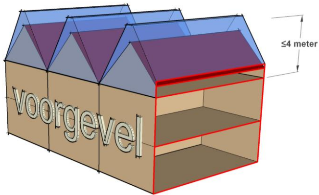
Aanzicht voorzijde "dwarskap" Kapprofiel A: \leq 55^\circ en \leq 4 m hoog
