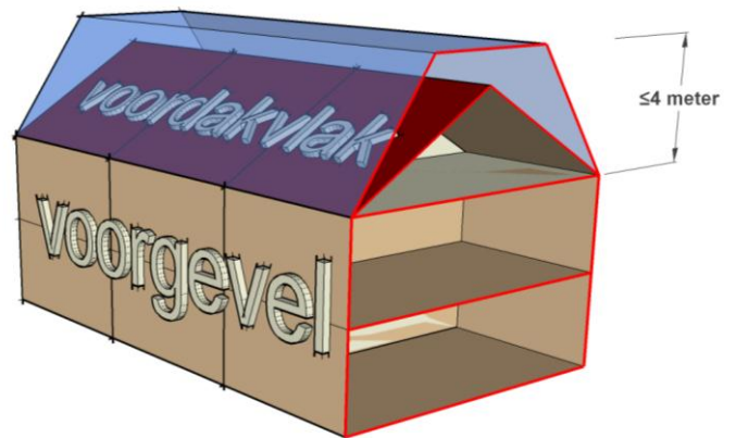
Aanzicht voorzijde "langskap" Kapprofiel A: \leq 55^\circ en \leq 4 m hoog
