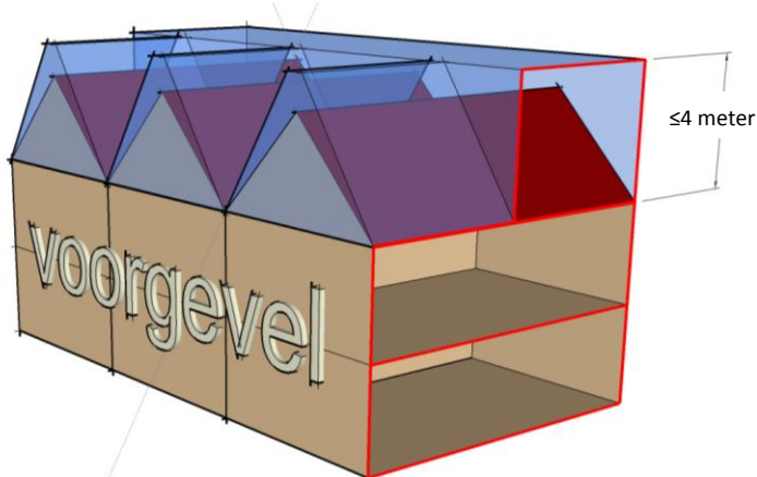
Aanzicht voorzijde "dwarskap" Kapprofiel B: \leq 55^\circ en \leq 4 m hoog & dakopbouw achterste helft
