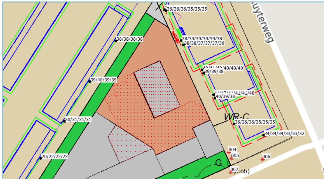
Afbeelding 5.3: overzicht maatgevende resultaten langtijdgemiddelde beoordelingsniveau ( L_{Ar,LT} ) inclusief stemgeluid, zonder het ophalen van afval
