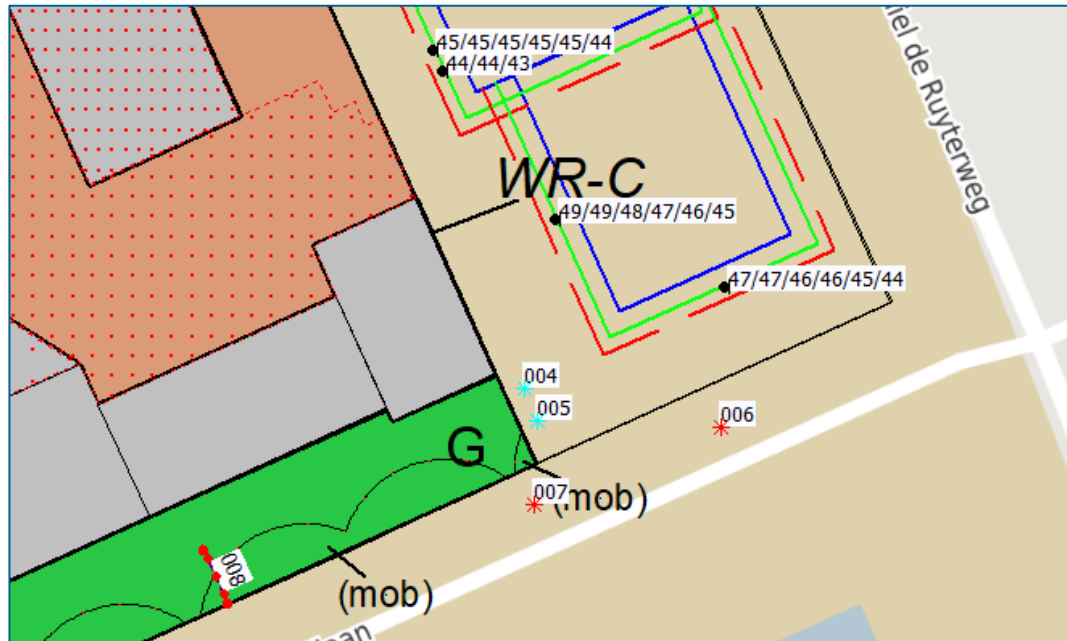
Afbeelding 5.2: overzicht maatgevende resultaten langtijdgemiddelde beoordelingsniveau ( L_{Ar,LT} ) als gevolg van alleen het ophalen van afval (bronnen 004 en 005)
