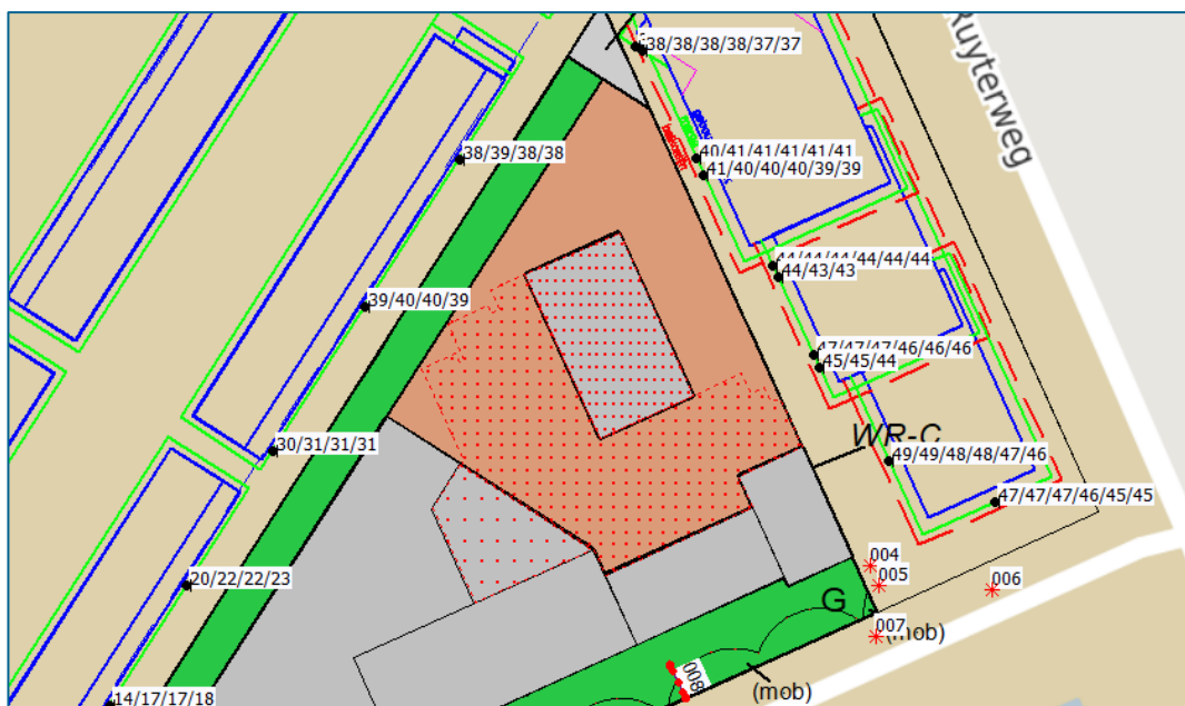
Afbeelding 5.1: overzicht maatgevende resultaten langtijdgemiddelde beoordelingsniveau ( L_{Ar,LT} )
