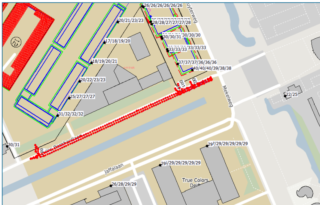
Afbeelding 5.4: overzicht maatgevende resultaten langtijdgemiddelde beoordelingsniveau ( L_{Ar,LT} )
