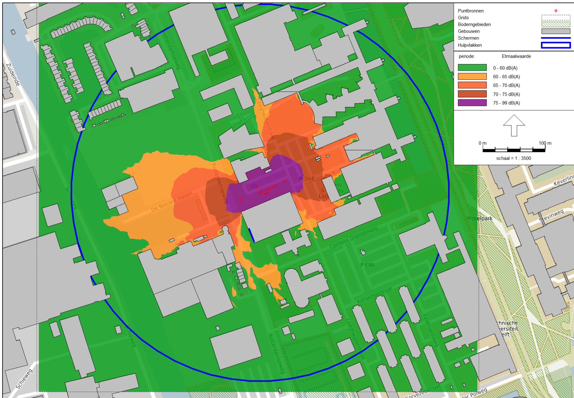
Figur 8 Geluidcontouren met bebouwing, 5m hoogte.
