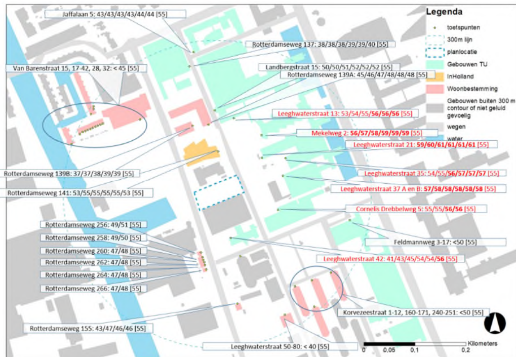
Afbeelding 3.2 Geluidniveaus in de avond op geluidgevoelige gebouwen met steeds van links naar rechts de berekende waarden op verschillende oplopende hoogtes en tussen vierkante haken de toetsingswaarde.
