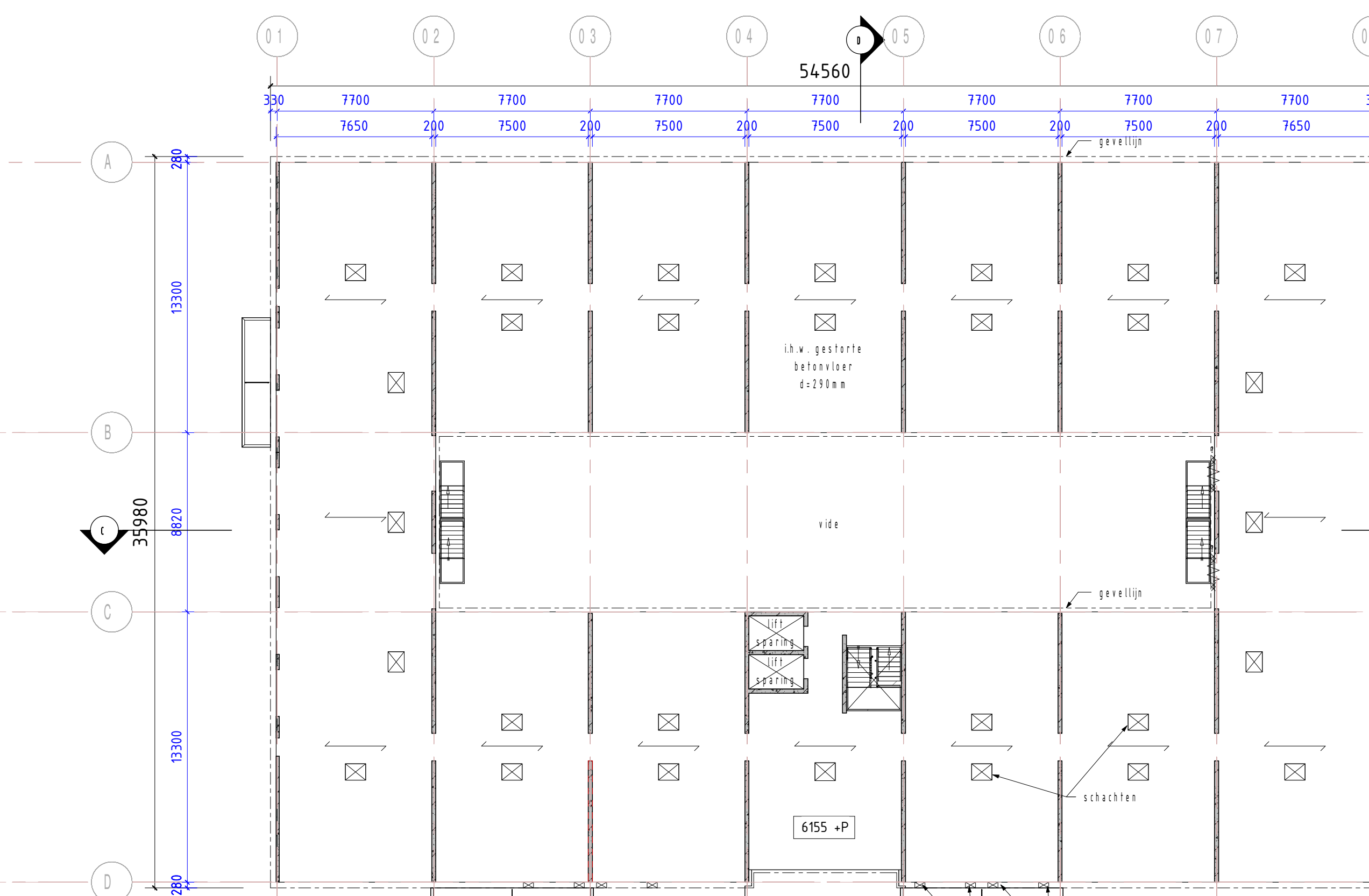
2e t/m 5e verdieping (voor balkon posities zie gevels)
