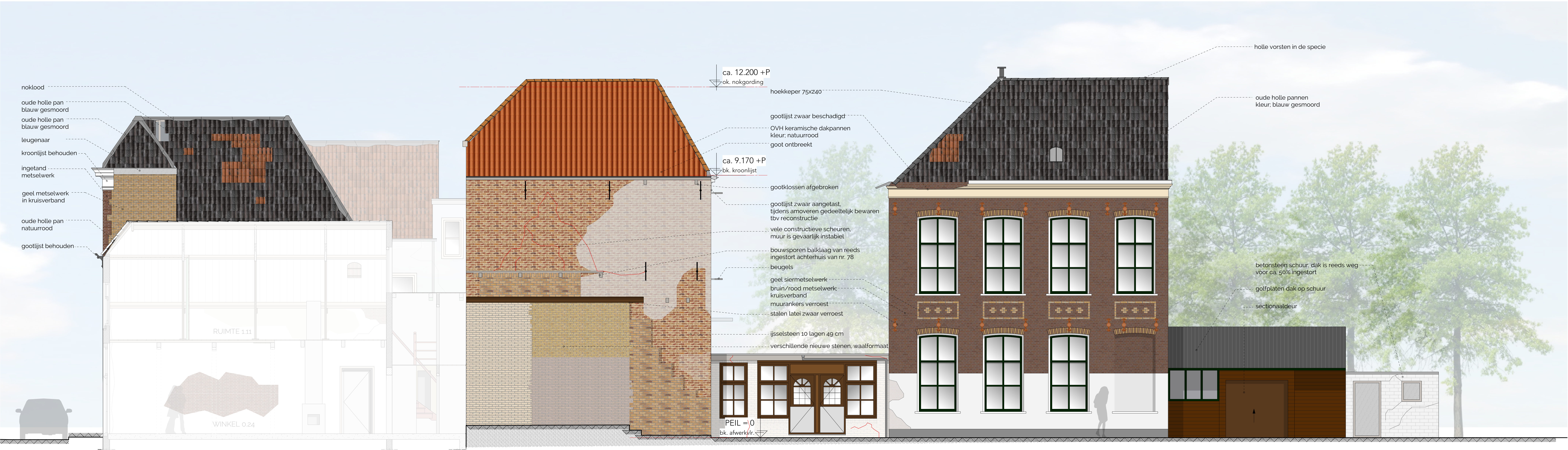
Doorsnede H-H - rechter zijgevels schaal 1:50
