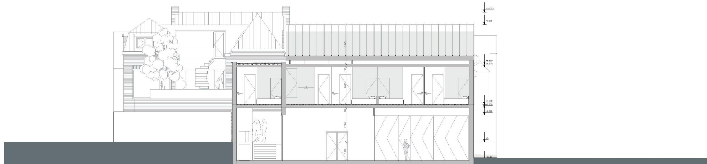
DOORSNEDE EE NIEUW
