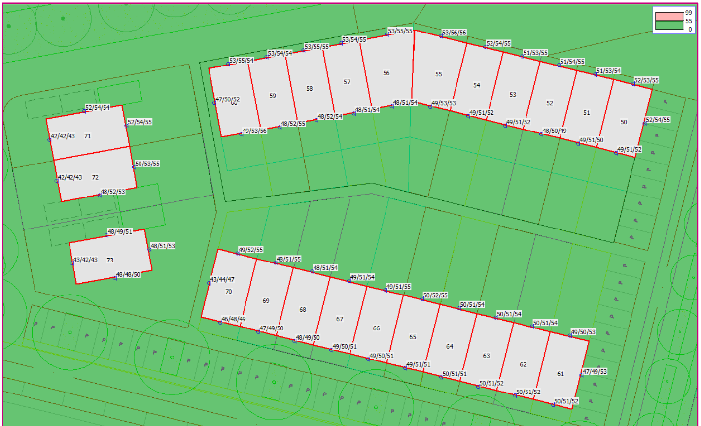
Figuur 5.19 Rekenresultaten industrielawaai objecten 50t/m 73, geluidcontour op 1,5 m
