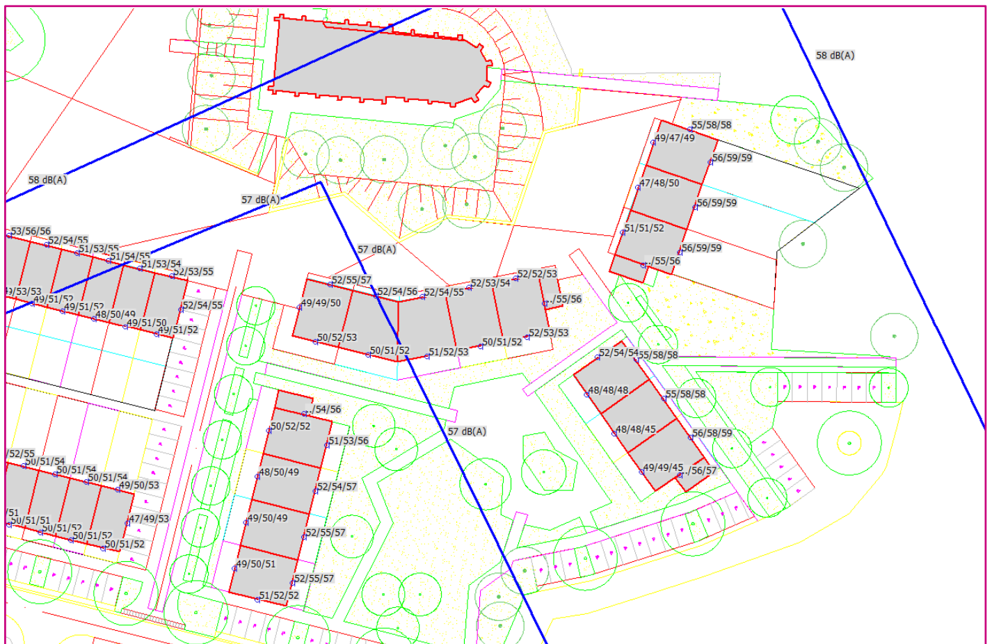
Figuur 5.3 Overzicht van rekenresultaten industrielawaai ten opzichte van RAK contouren
