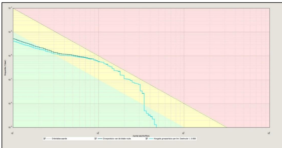
Figuur 6.1: fN-curve autonome situatie
