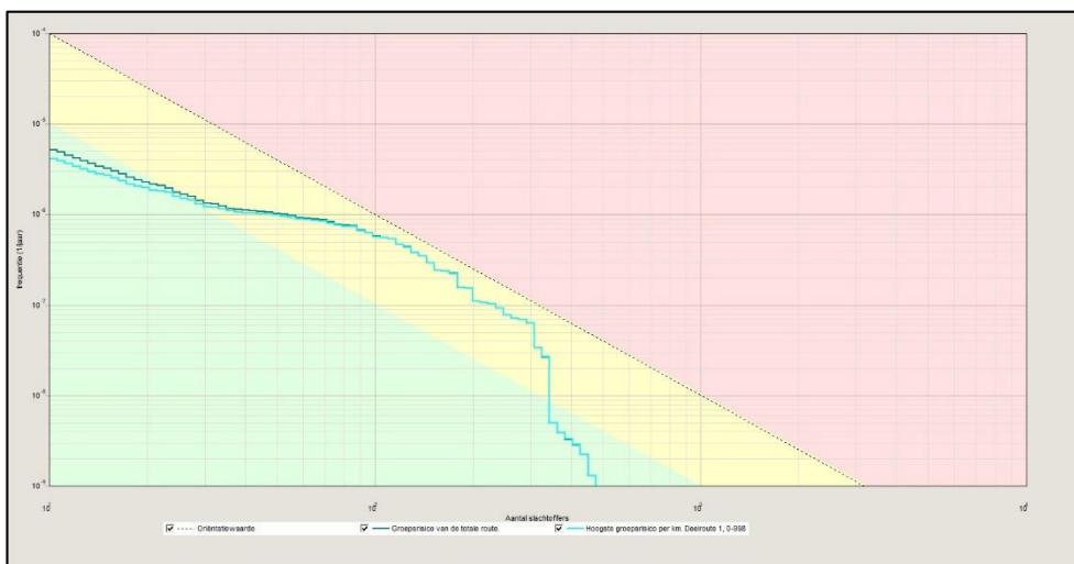
Figuur 6.2: fN-curve toekomstige situatie
