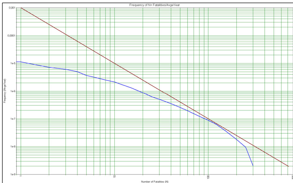
Figuur 4.2: fN-curve Rangeerterrein Kijfhoek
