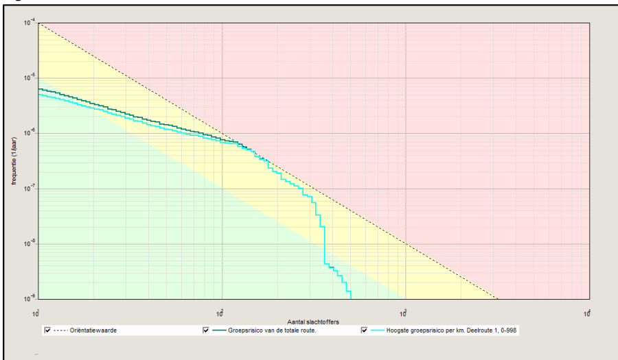
Figuur 4.1: fN-curve autonome situatie
