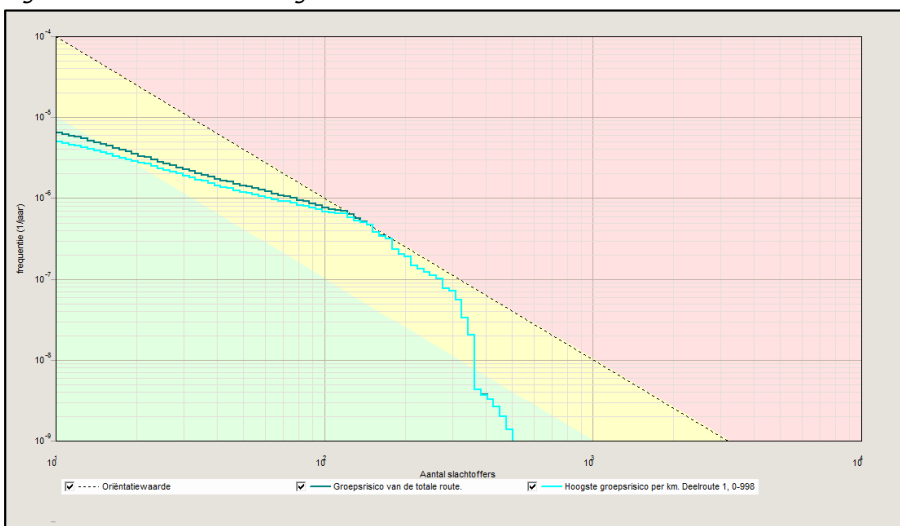
Figuur 4.2: fN-curve toekomstige situatie
