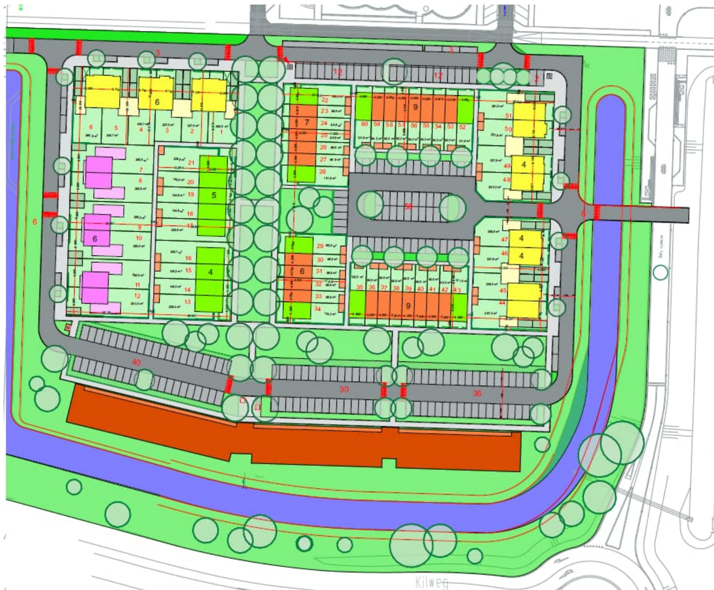
Figuur 2-7 Verkavelingsopzet
