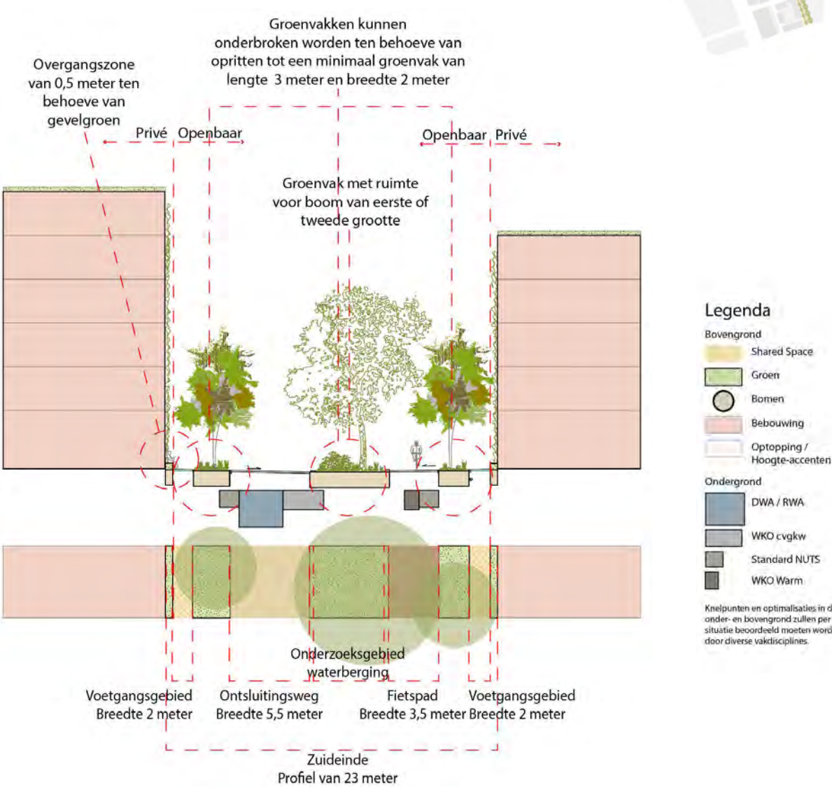
Doorsnede Zuideinde 2
