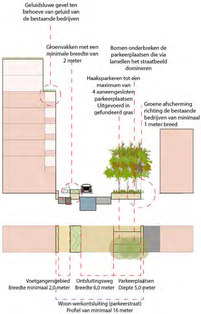
Doorsnede Parkeerstraat 1
