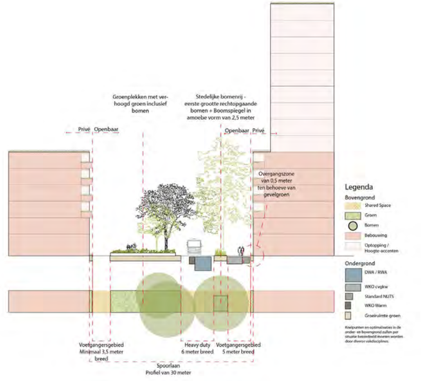
Doorsnede 2: Spoorlaan
