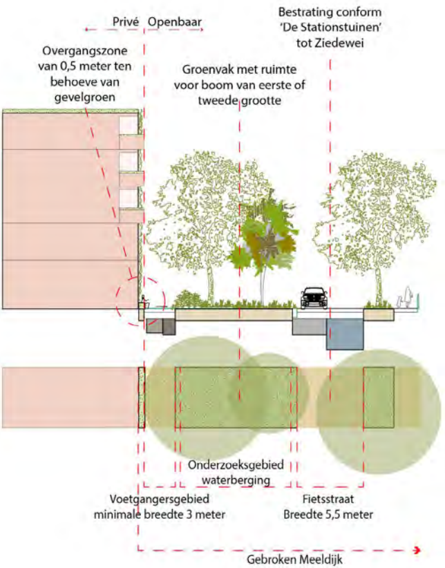
Doorsnede Gebroken Meeldijk 1
