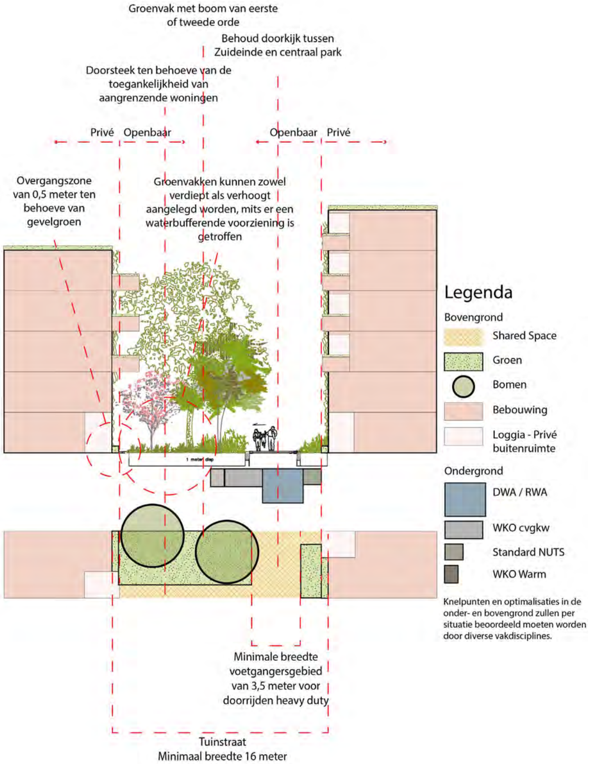
Doorsnede 1: Tuinstraat
