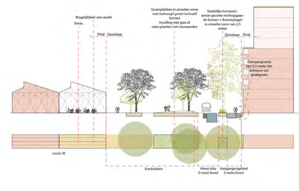
Doorsnede 1: Plein Loods 38
