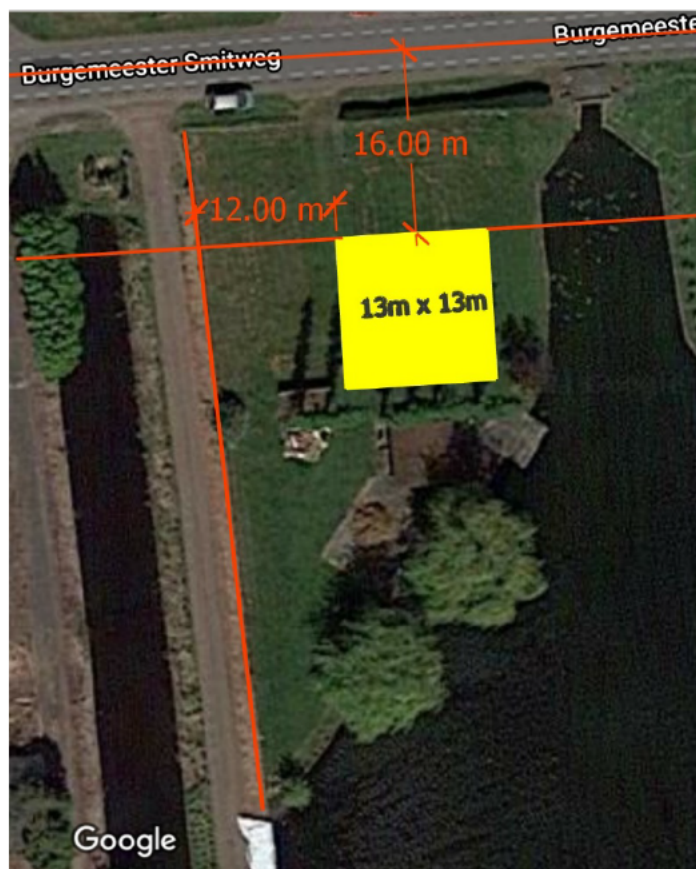
Figuur 1: Situatieschets bouwvlak Burgermeester Smitweg tussen 17 en 19
