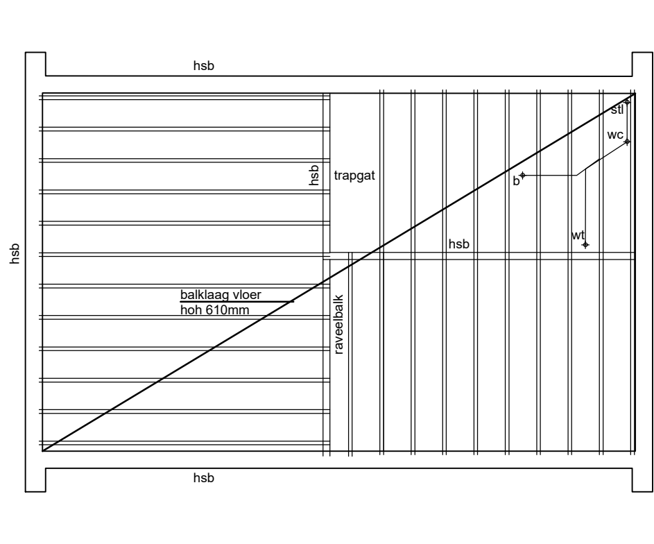
principe 1e verdiepingsvloer
