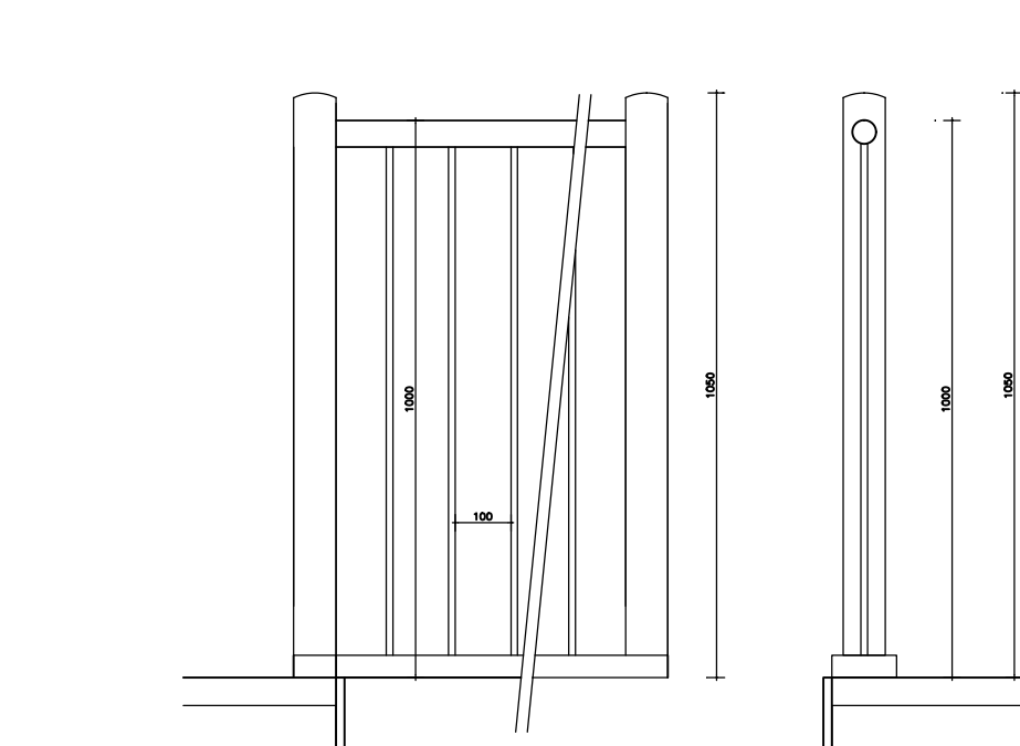
principe trap en baluster 1:30
