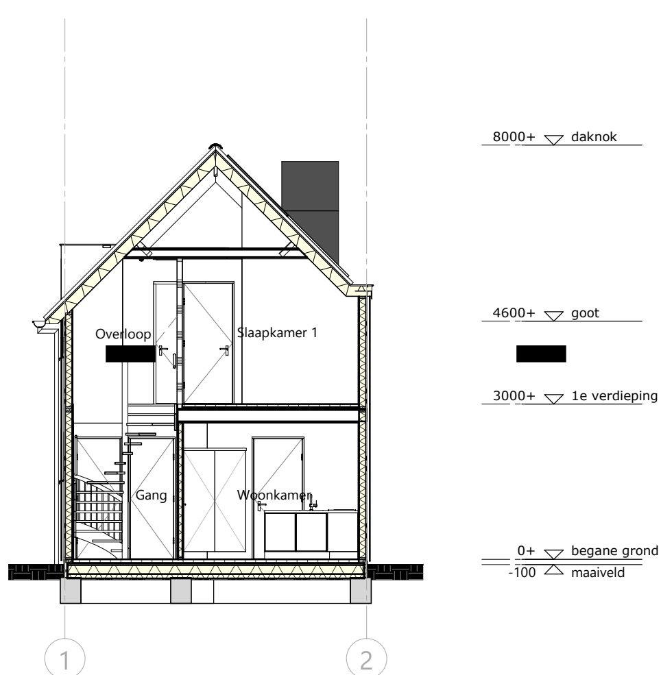
doorsnede A-A - 1 : 100
