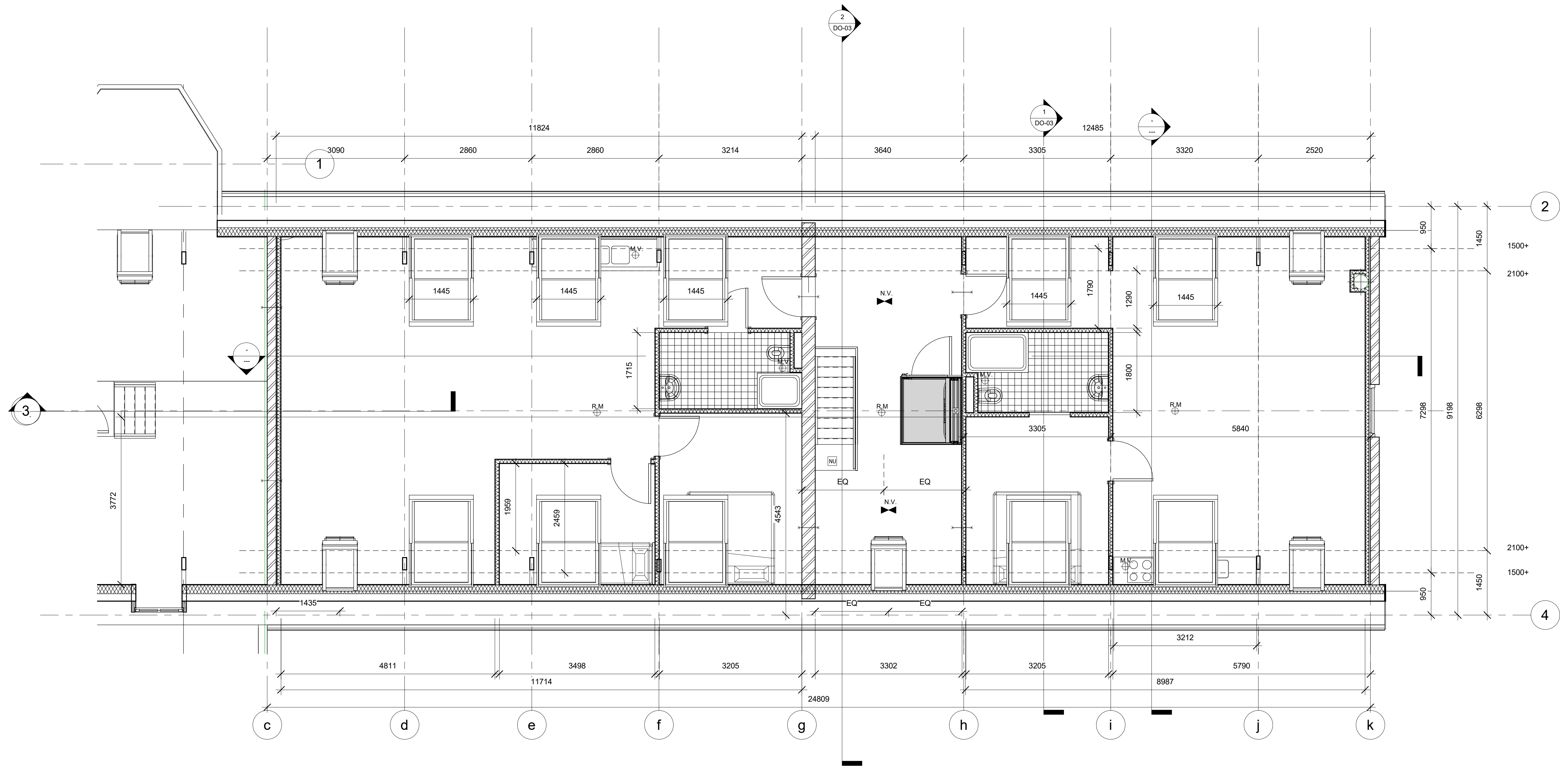
1 1e verdieping stal 1 : 50
