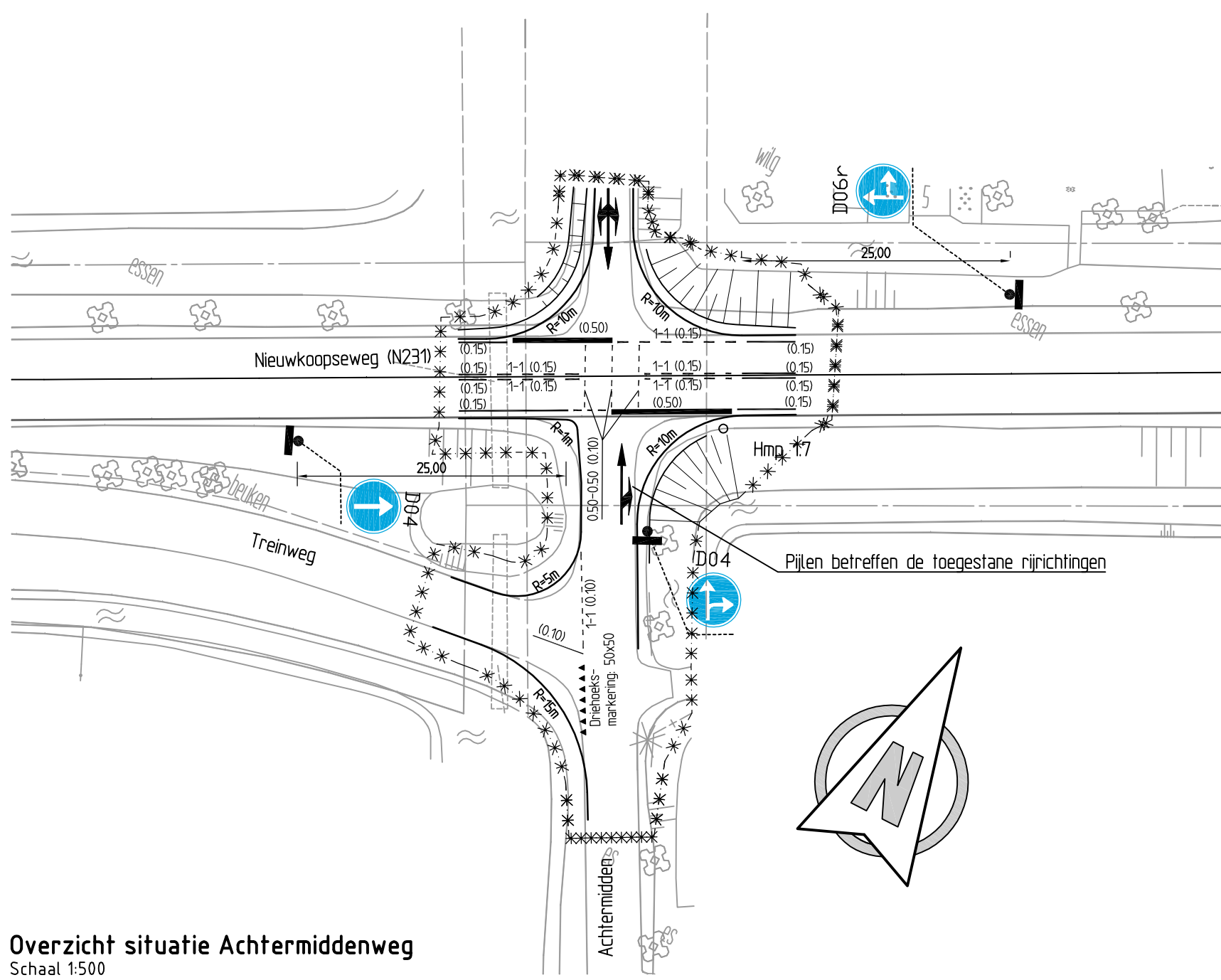
Overzicht situatie Achtermiddenweg Schaal 1:500
