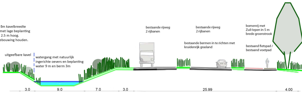
profiel Maximabrug Hoorn-West
