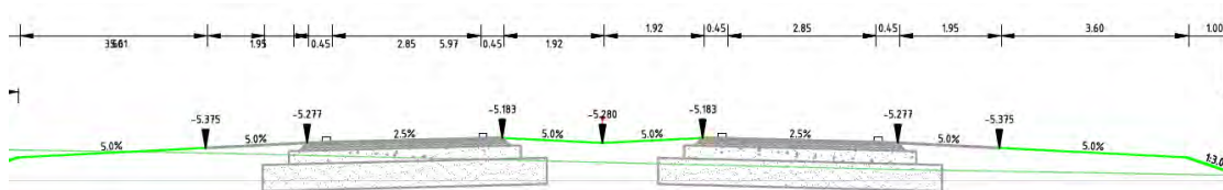
Figuur 22: doorsnede 10 Verlengde Bentwoudlaan metring 4250.000
