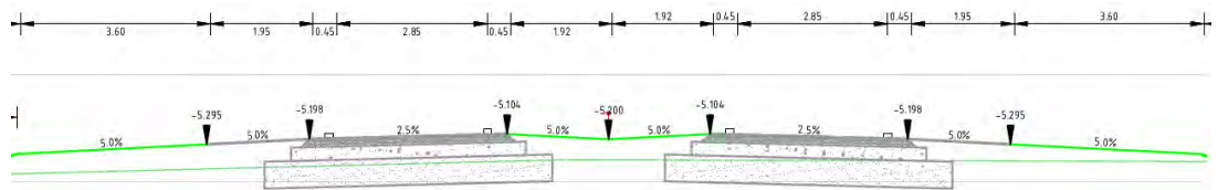
Figuur 19: dwarsdoorsnede 2 Bentwoudlaan
