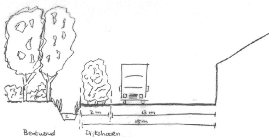
Afbeelding 5: Doorsnede erfscheiding ter hoogte van groene haag (inrichting Bentwoud is indicatief)
