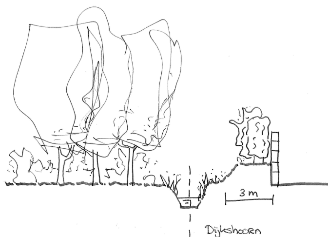
Afbeelding 8: Doorsnede erfscheiding ter hoogte van wal met beplanting oostzijde
