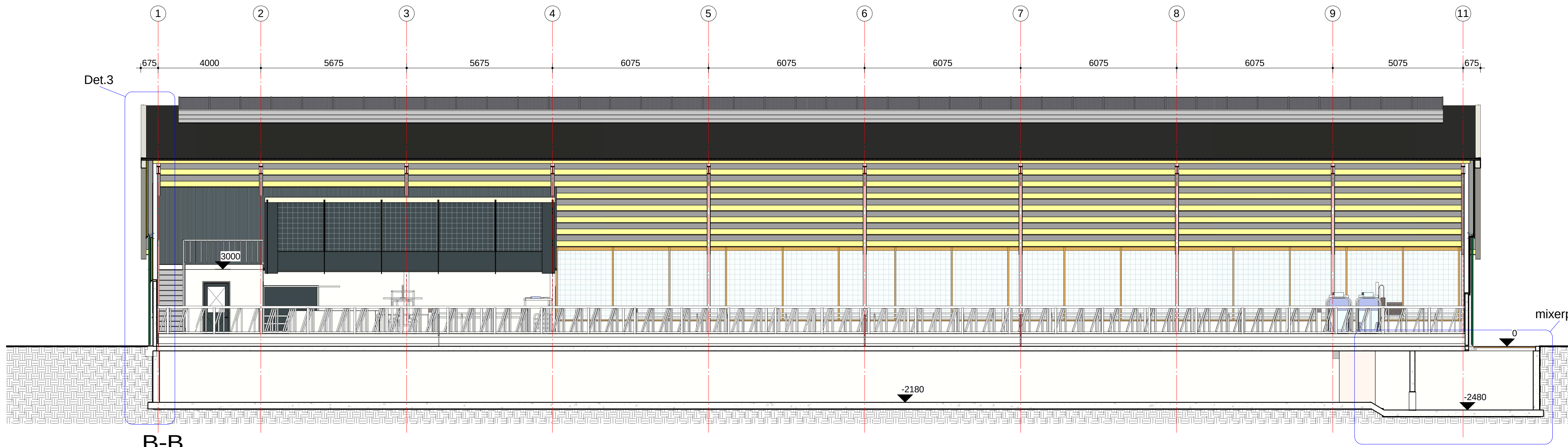
B-B
