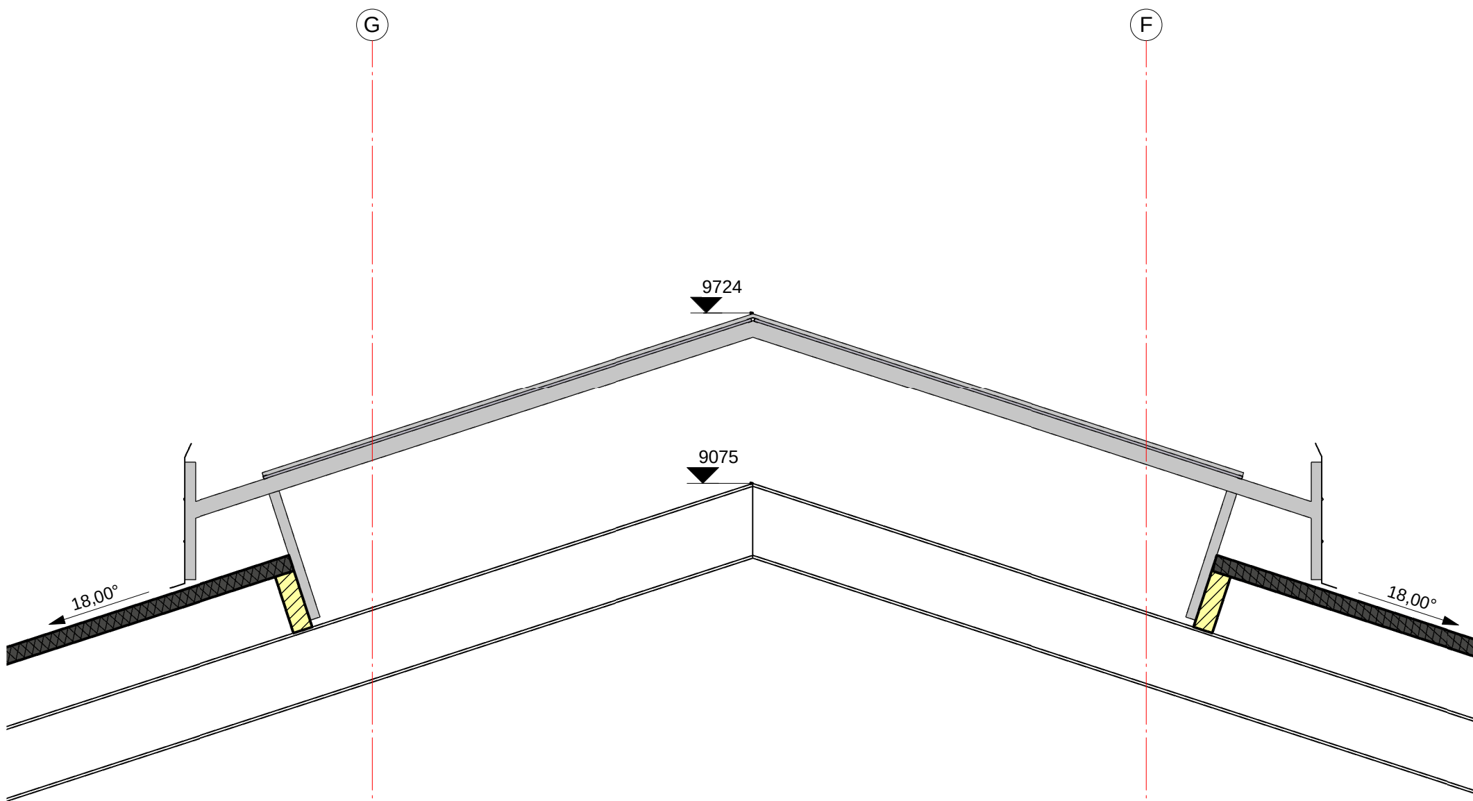
Det.2
