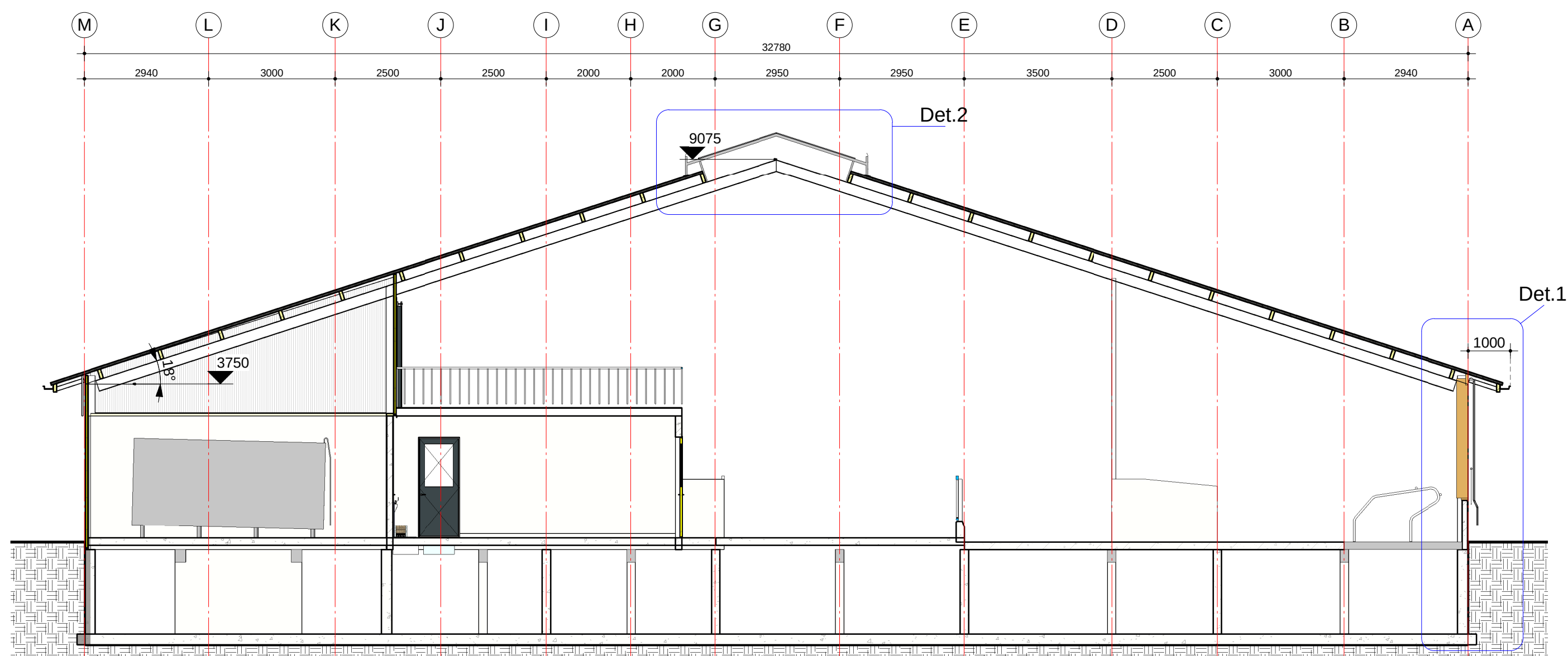
A-A
