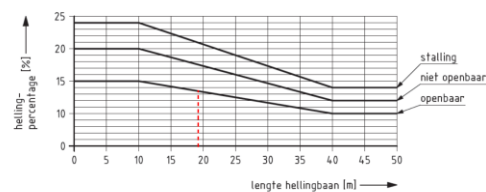
Figuur 36 — Maximale hellingpercentages per type parkeervoorziening
