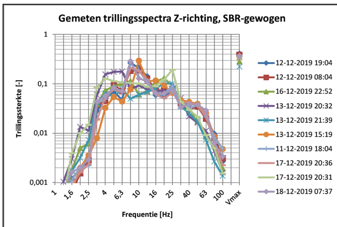
Figuur 5.1: Overzicht gewogen trillingsspectra treinpassages maaiveld zuid in prognose
