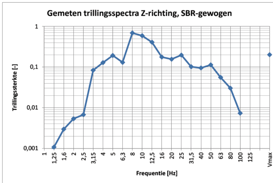
Figuur 4.2: Maxhold spectrum passage trein figuur 4.1
