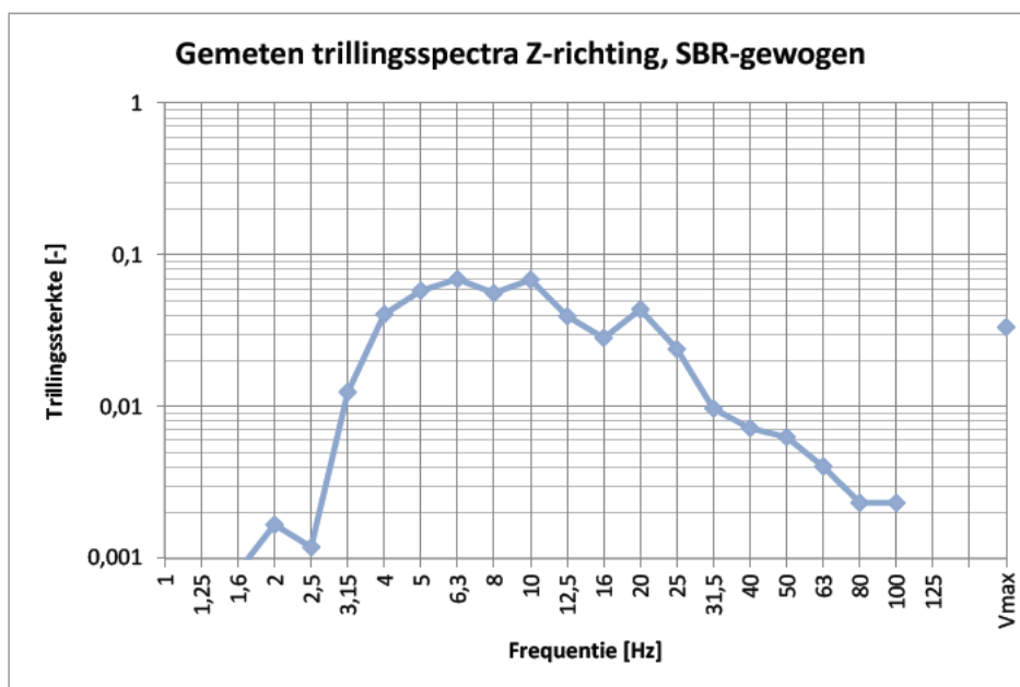
Figuur 4.4: Maxhold spectrum passage trein figuur 4.3
