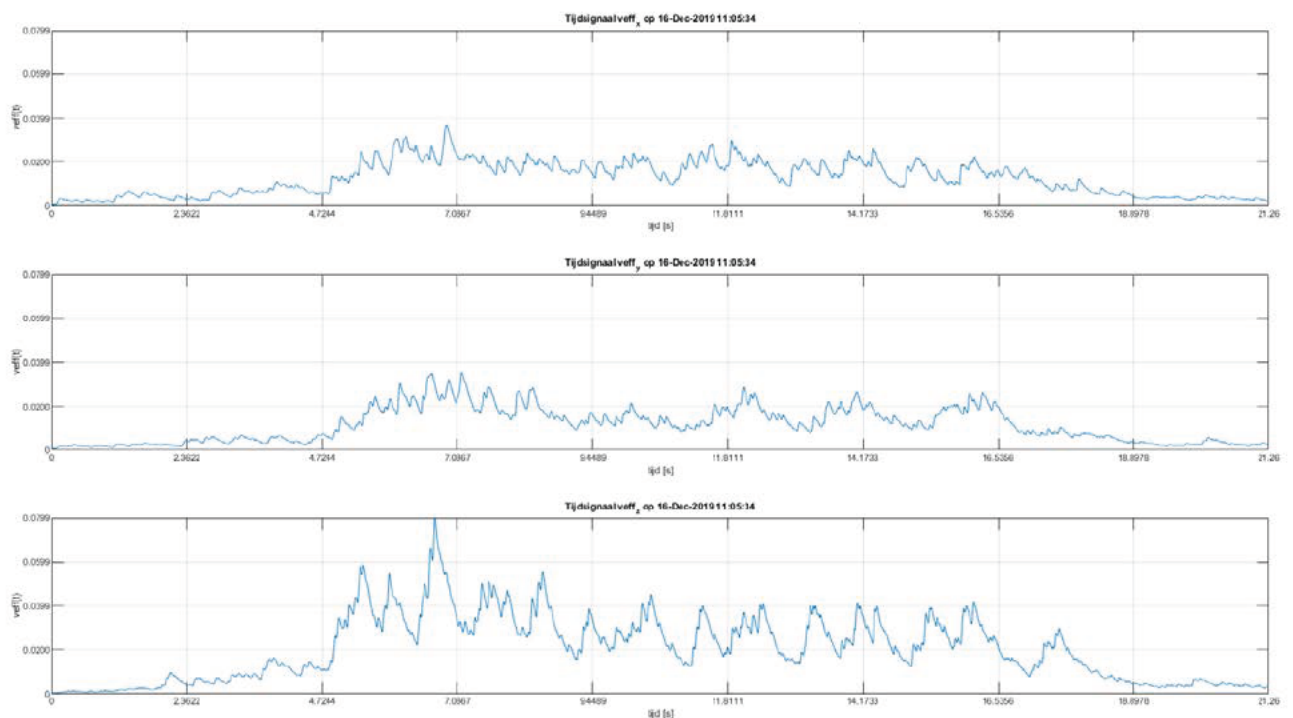
Figuur 4.3: Verloop voortschrijdende effectieve trillingssterkte treinpassage met hoogste V_{max} (fundering)
