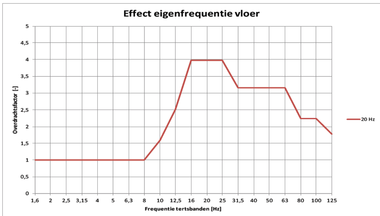
Figuur 5.3: Overdrachtsfactor vloer voor een eigenfrequentie van 20 Hz
