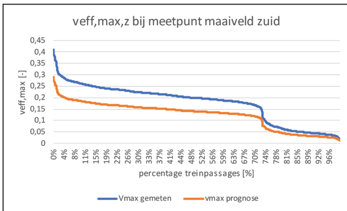
Figuur 5.4: Cumulatieve verdeling v_{\text{max}} per treinpassage voor meetpunt maaiveld zuid
