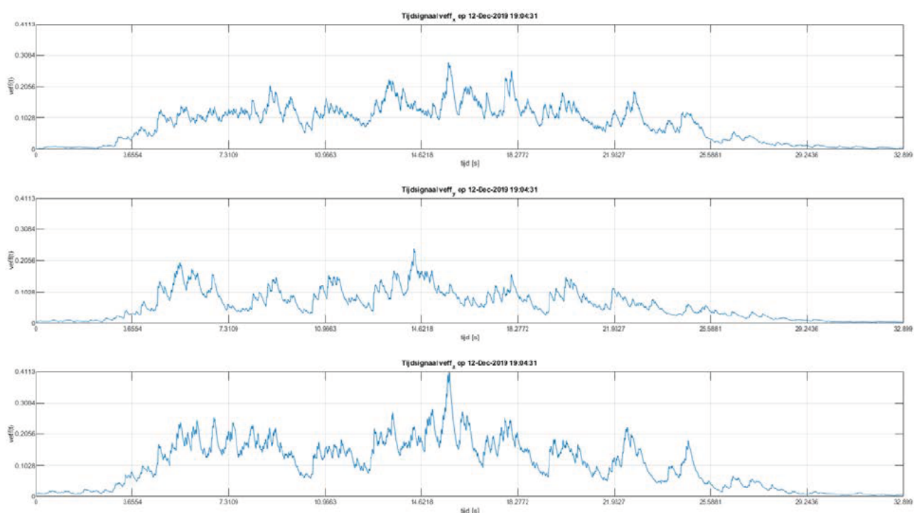
Figuur 4.1: Verloop voortschrijdende effectieve trillingssterkte treinpassage met hoogste V_{\max} (maaiveld aan de zuidkant)
