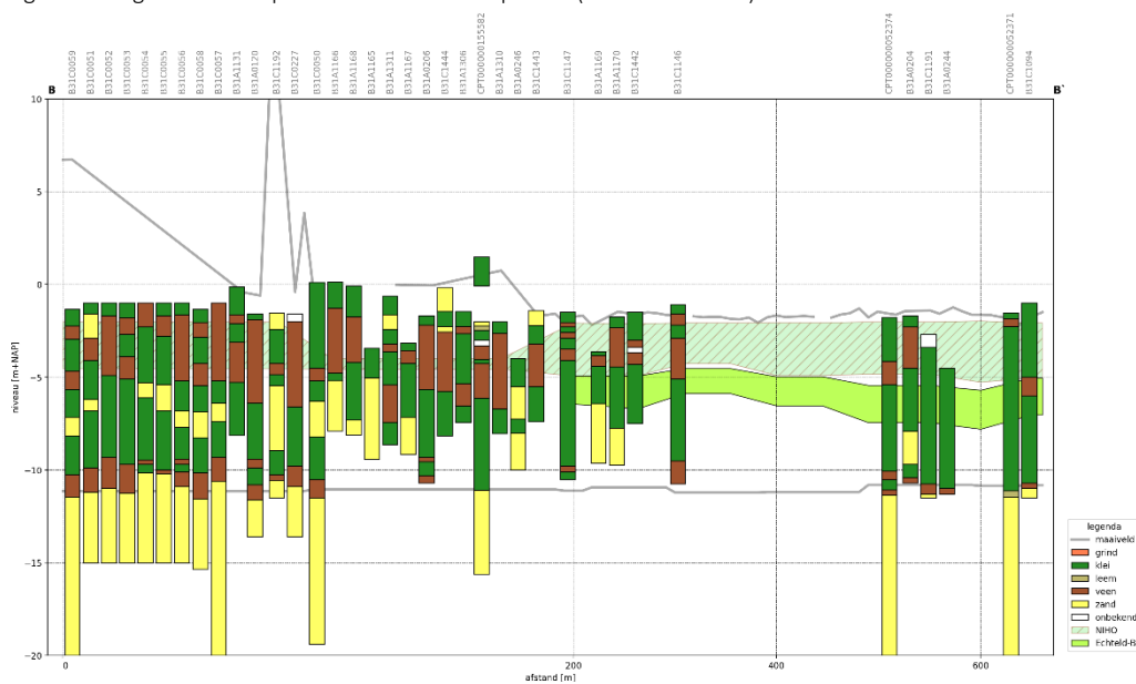
Figuur 2.11: globaal dwarsprofiel van de bodemopbouw (Bron: DINoloket)
