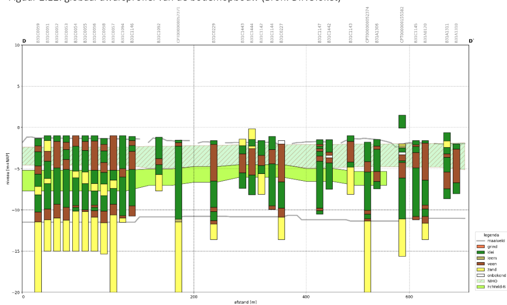
Figuur 2.13: globaal dwarsprofiel van de bodemopbouw (Bron: DINOLOket)
