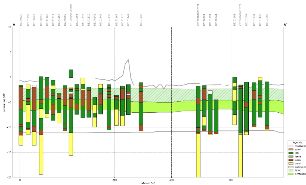
Figuur 2.10: globaal dwarsprofiel van de bodemopbouw (Bron: DINoloket)
