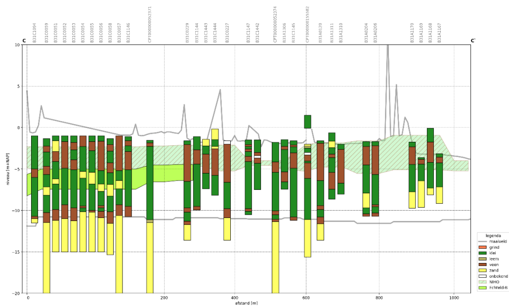
Figuur 2.12: globaal dwarsprofiel van de bodemopbouw (Bron: DINOLOket)
