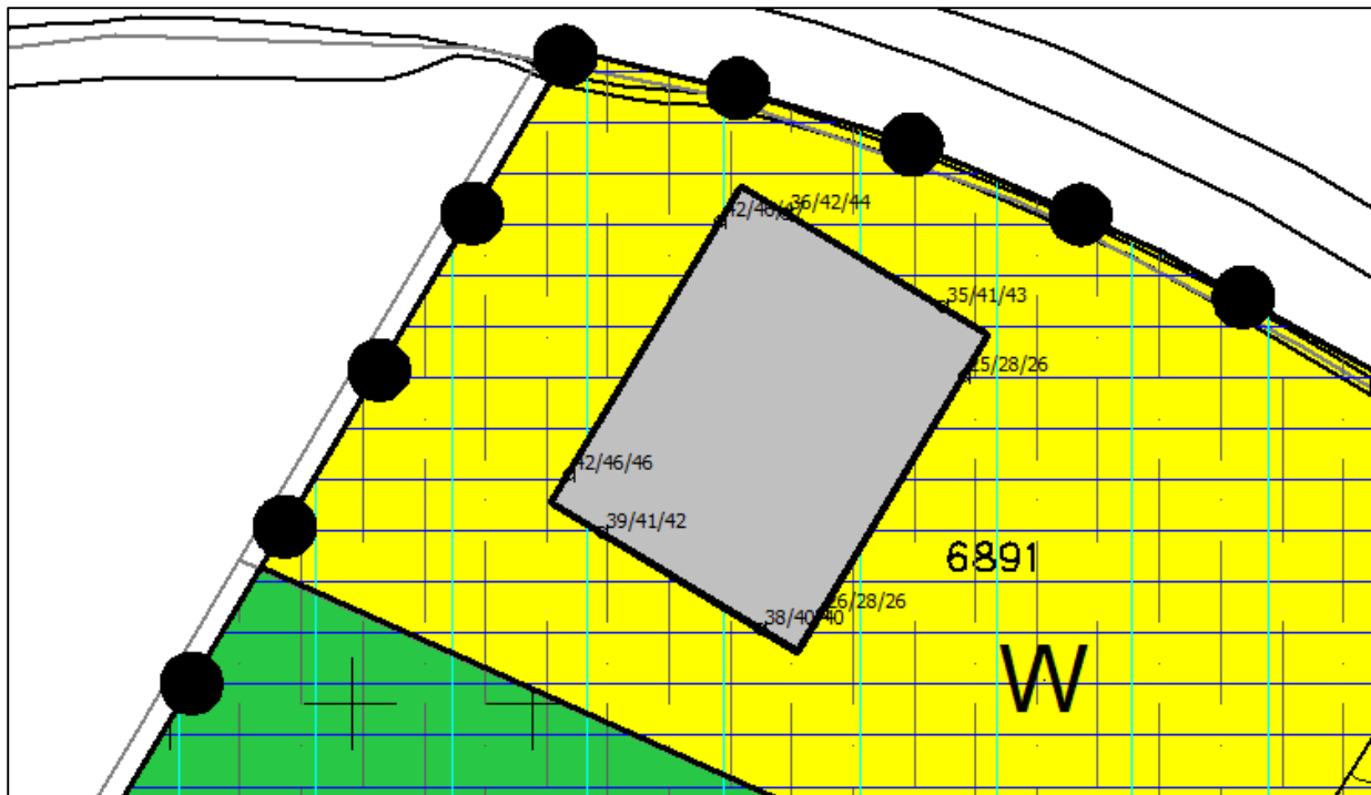
Figuur 6: Geluidsbelastingen afkomstig van de Paltrokmolen
