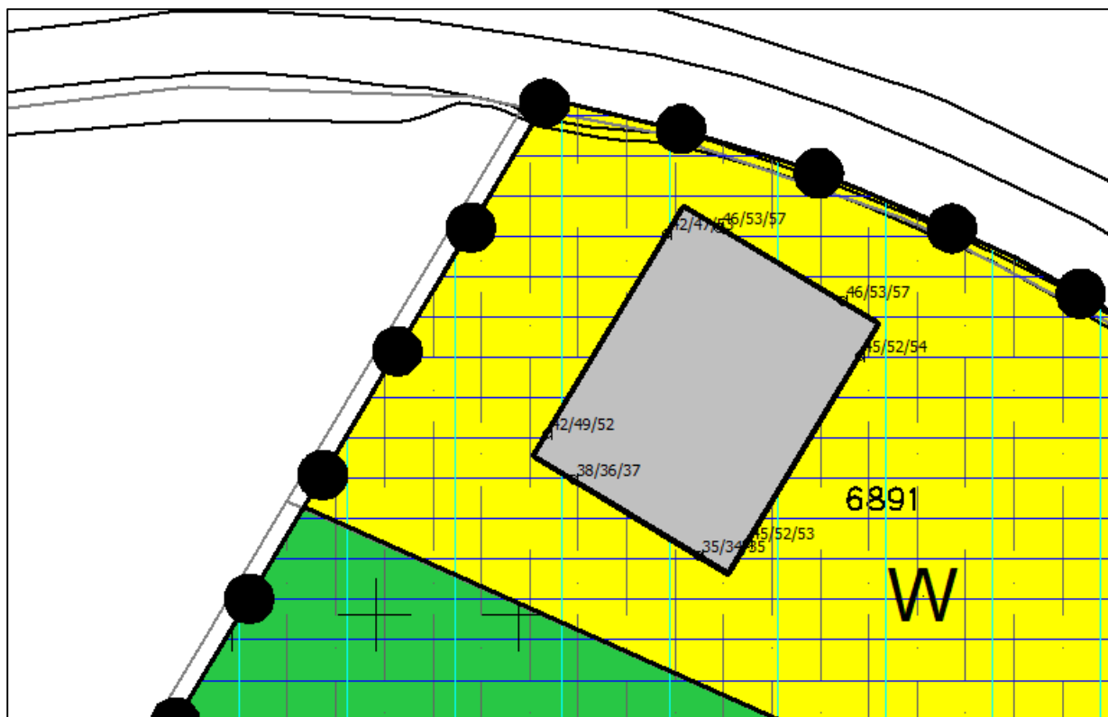
Figuur 4: Geluidsbelastingen afkomstig van de Oranje Nassausingel
