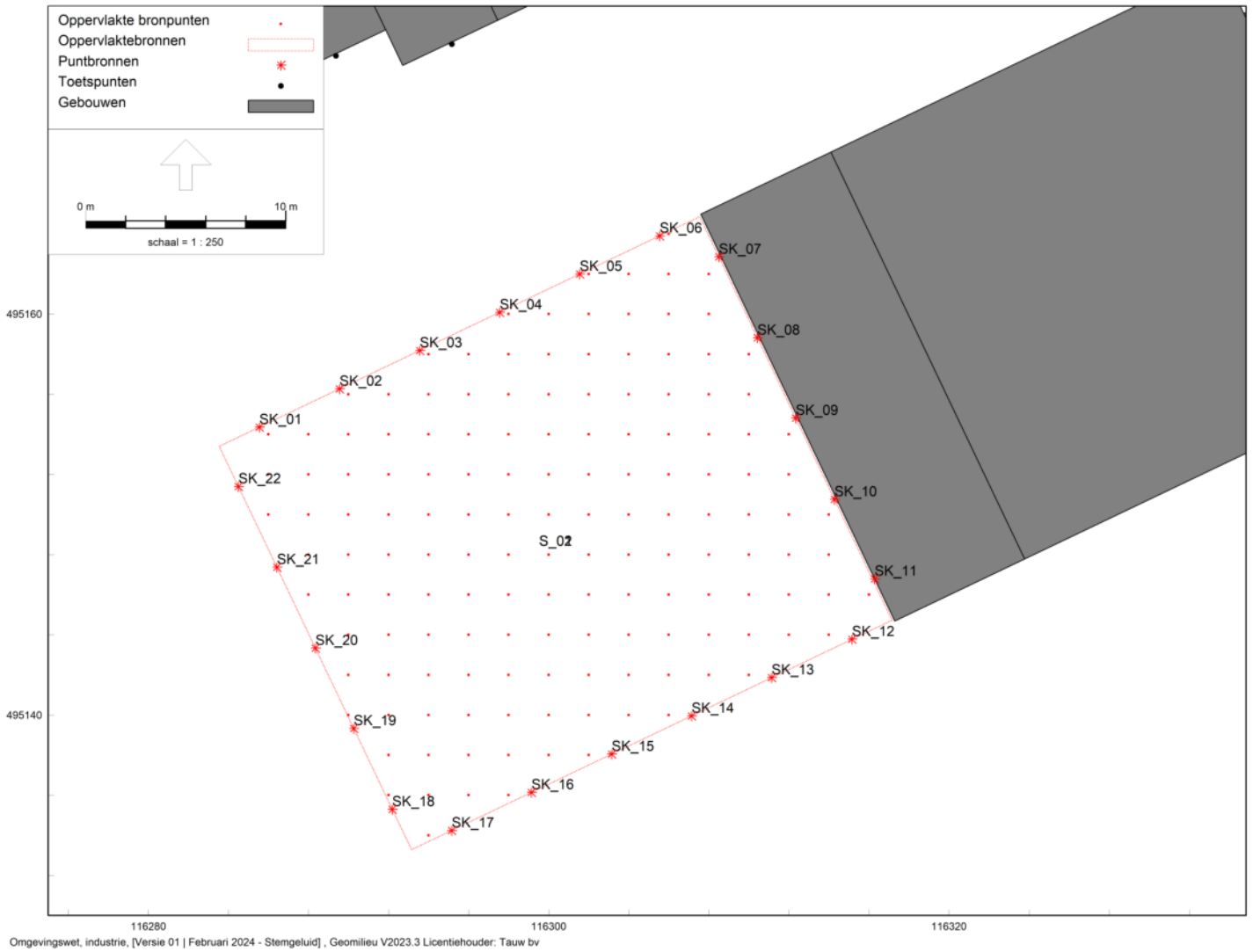
Figuur 3 | Overzicht rekenmodel met identificatie oppervlakte- en puntbronnen
