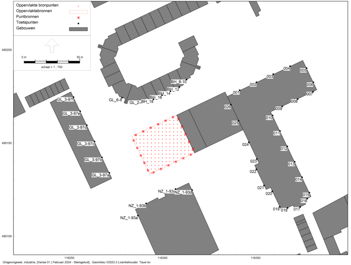
Figuur 2 | Overzicht rekenmodel met identificatie toetspunten
