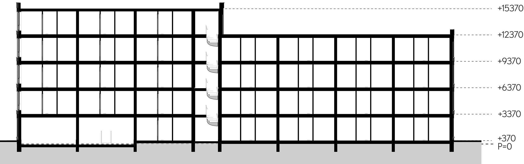
Doorsnede (1:200)
