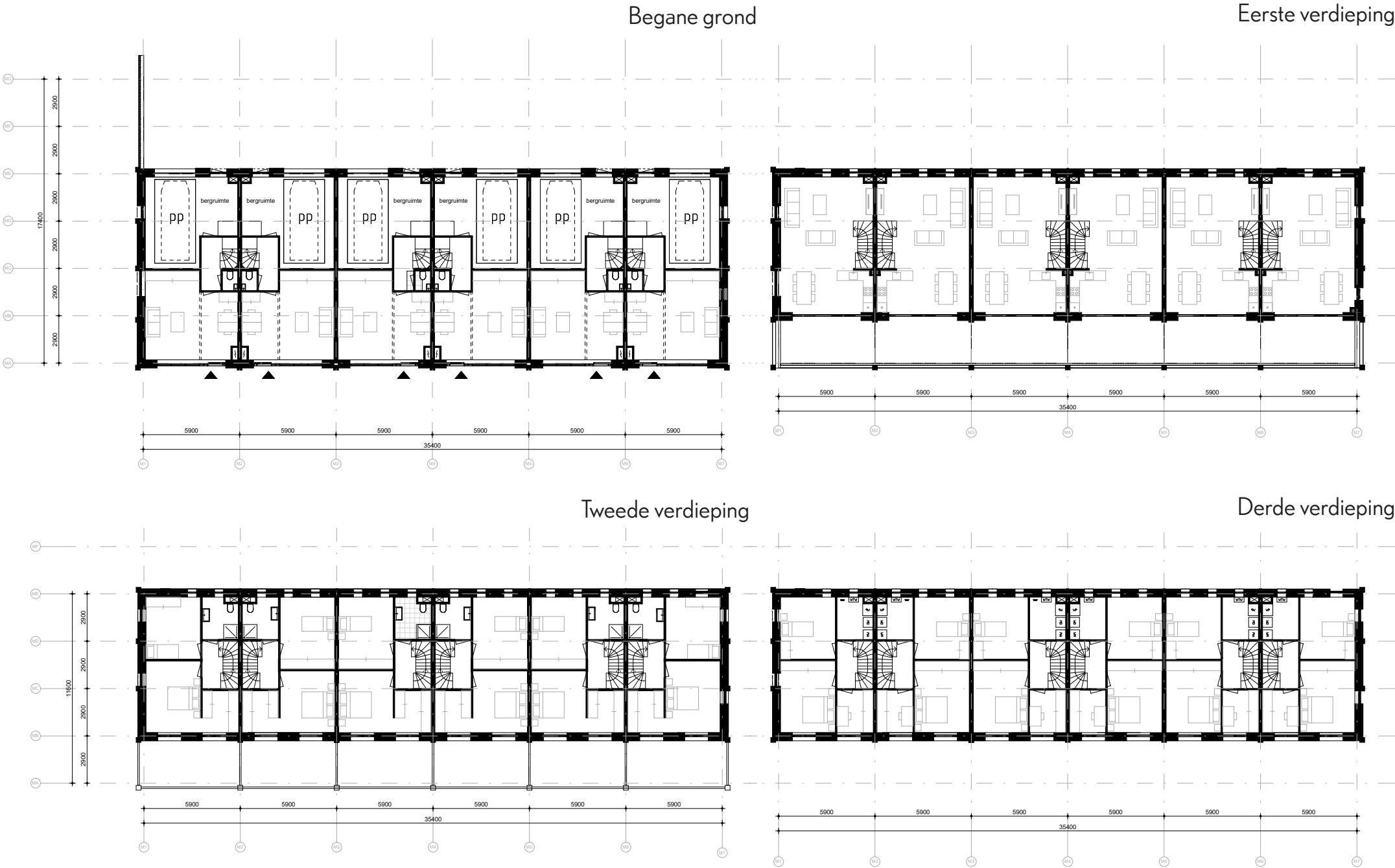
Plattegronden
