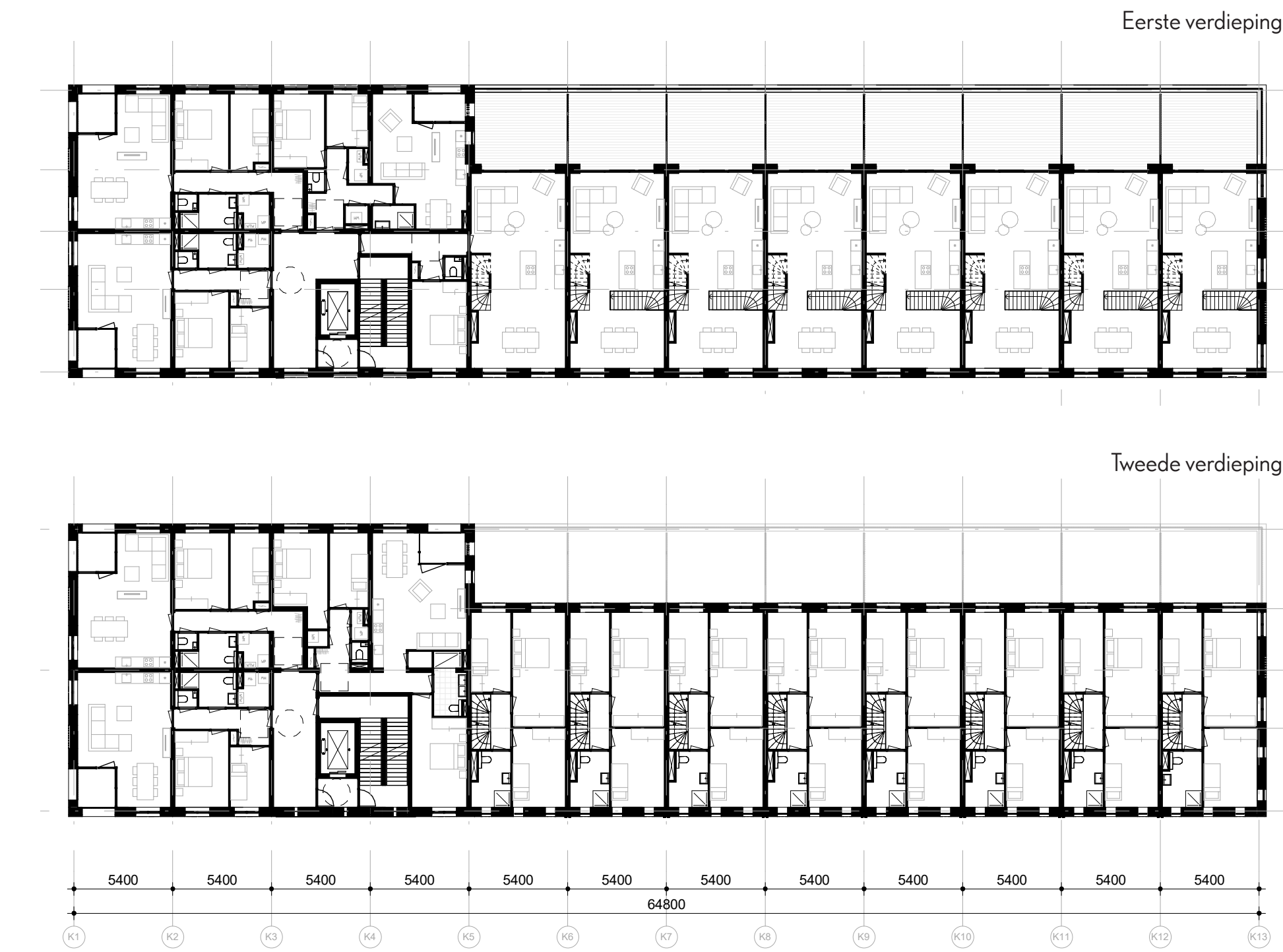
Plattegronden
