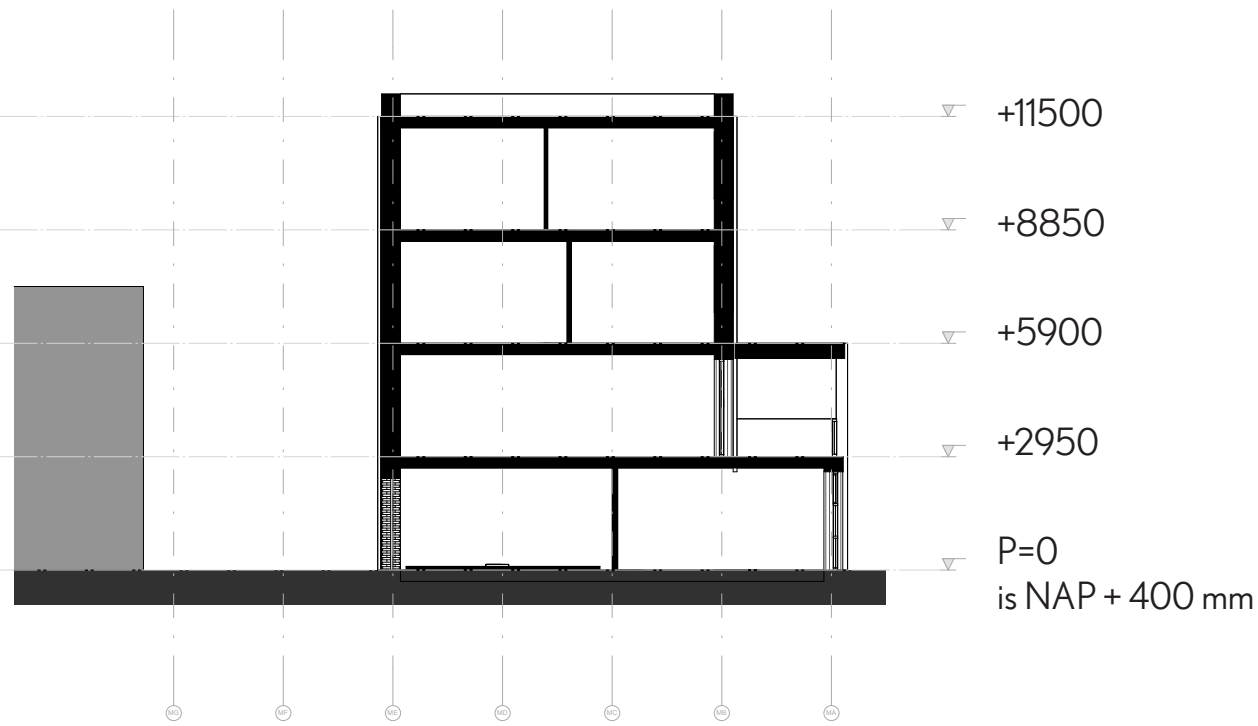
Doorsnede noord-zuid
