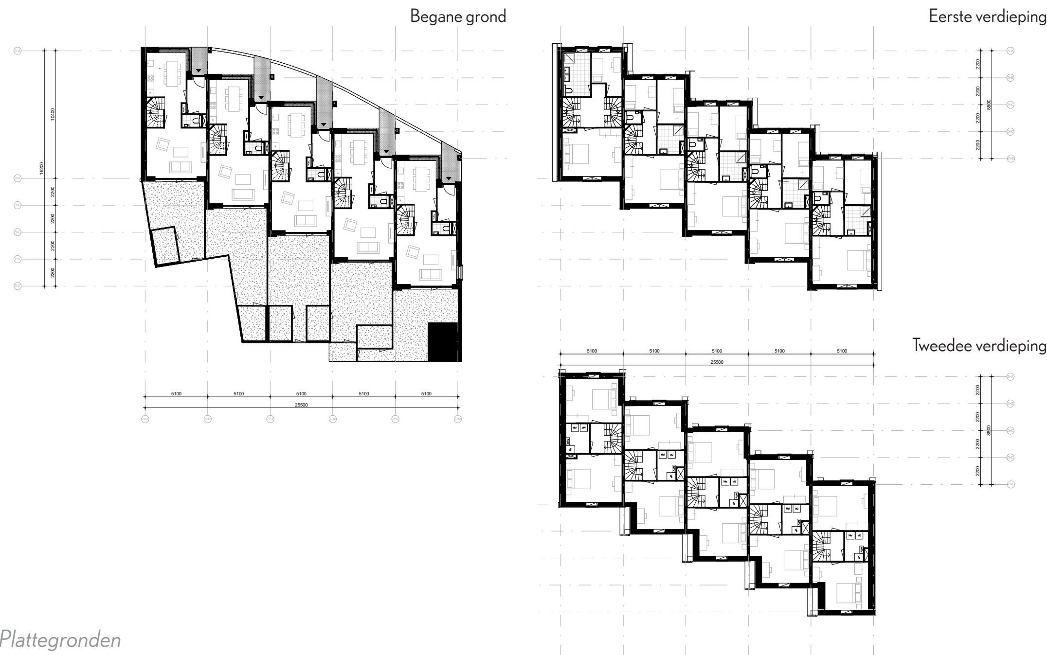
Plattegronden
