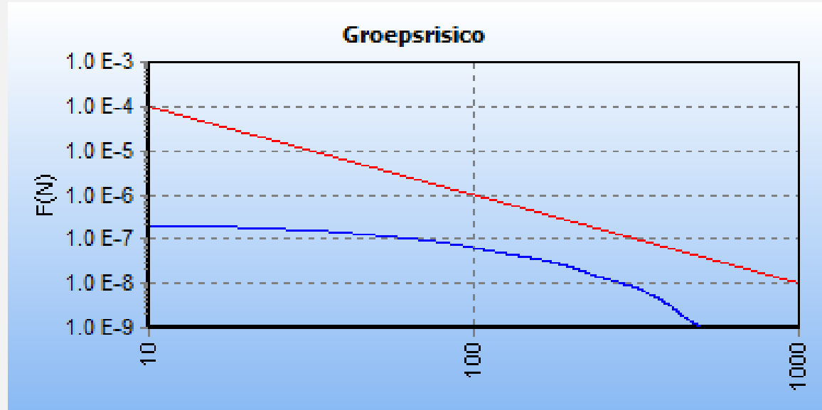
Figuur 6.3 FN curve voor buisleiding W-572-01 van Gasunie voor de kilometer tussen stationing 4730.00 en 5730.00 (bestaande situatie) en stationing 4320.00 en 5320.00 (nieuwe situatie)
