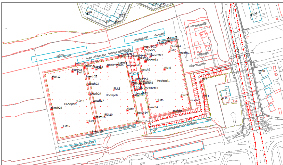
Figuur 2.4 Rekenmodel wedstrijddagen in 2D
