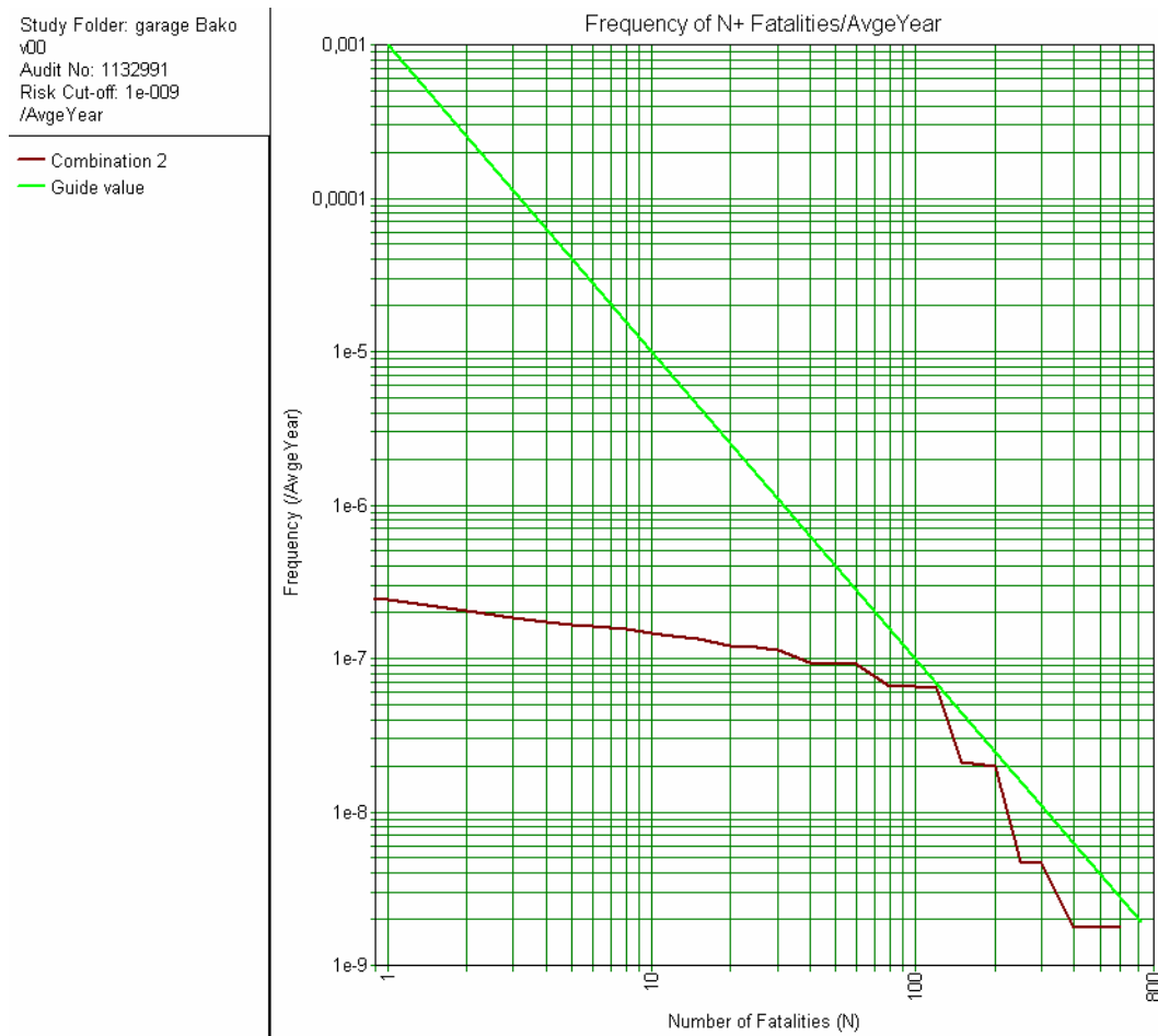
Figuur 4.1 Berekende groepsrisico
