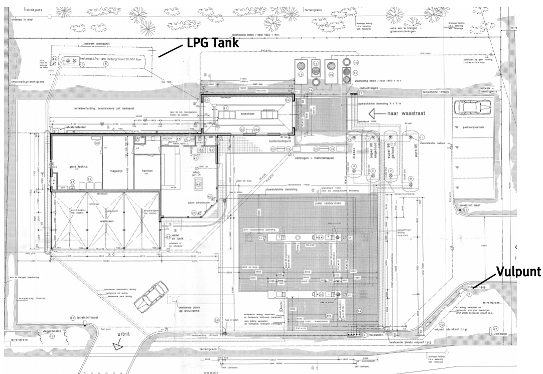
Figuur 2.2 Plattegrond LPG-tankstation "Garage Bako"
