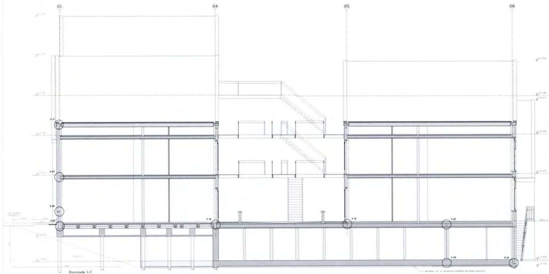
Doorsnede C-C
