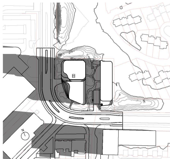
21 maart 9:00 1 : 2000
