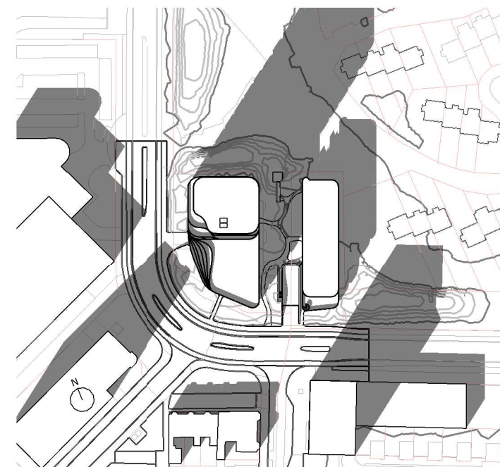
21 maart 16:00 1 : 2000
