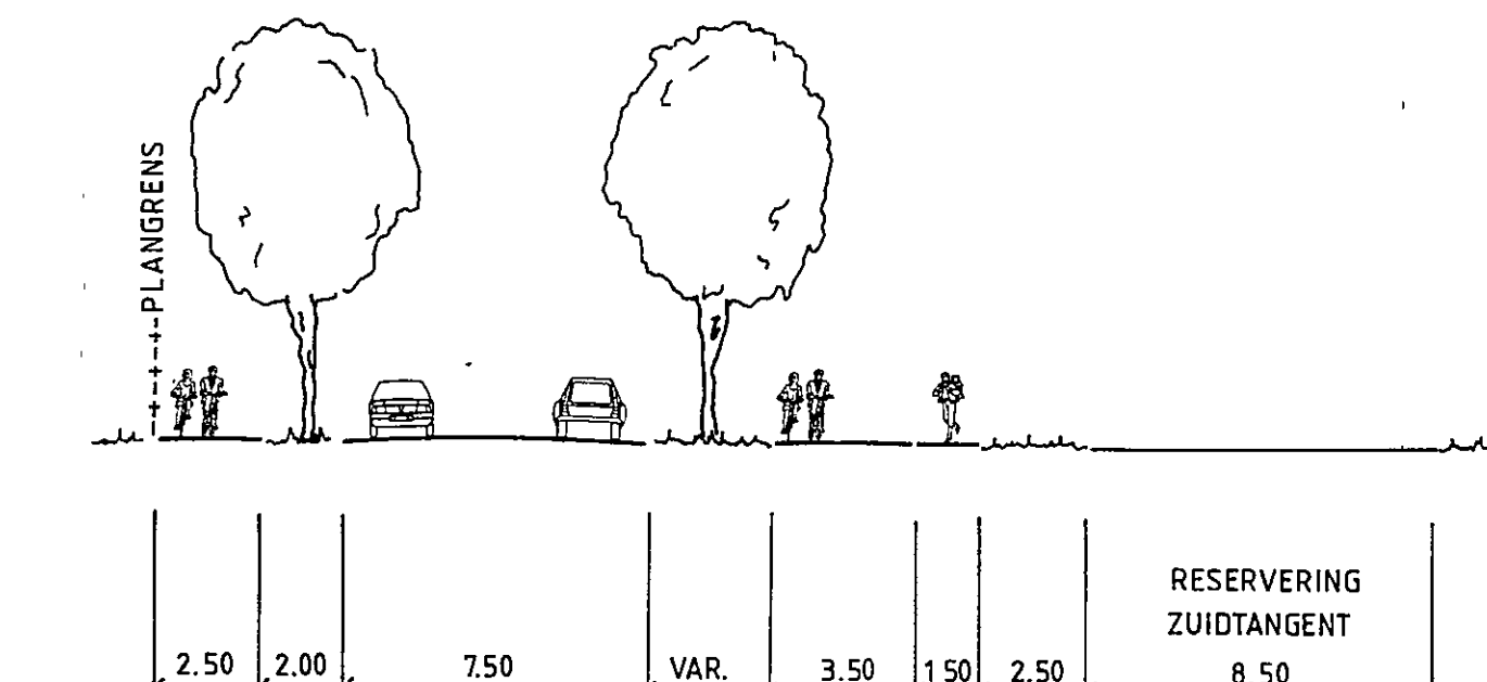
PROFIEL 1 Schaal 1:200
