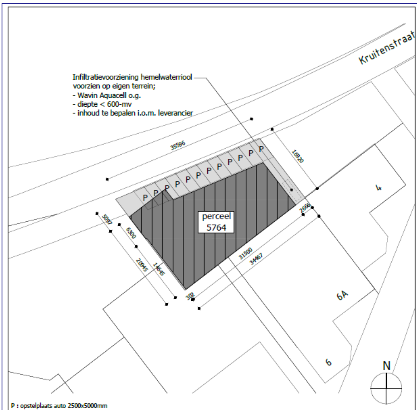
Situatie - Schaal 1:500
