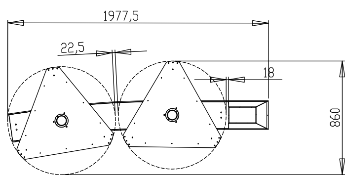
doorsnede B-B
