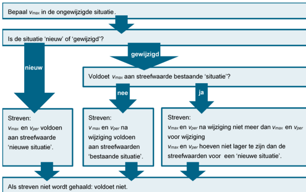
Figuur 2 Schematisatie beoordeling trillingen richtlijn Trillingen deel B
