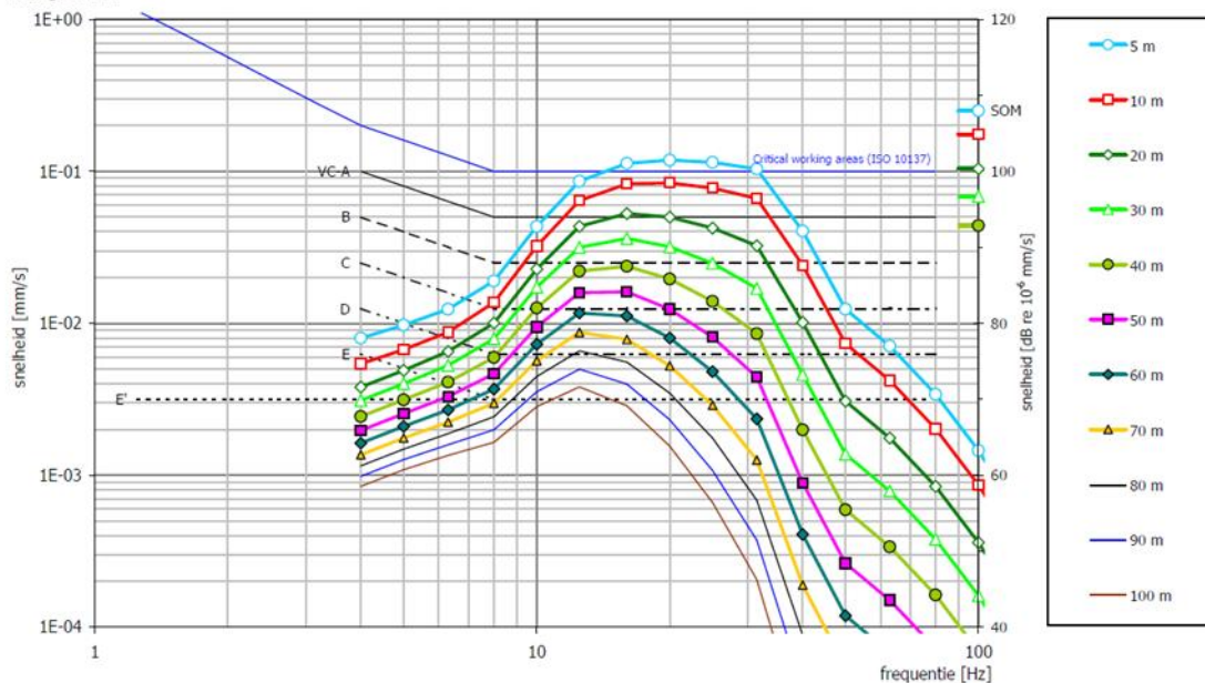
Figuur 3 Verwachtingswaarden trillingen lightrail (bron: ref[5])
