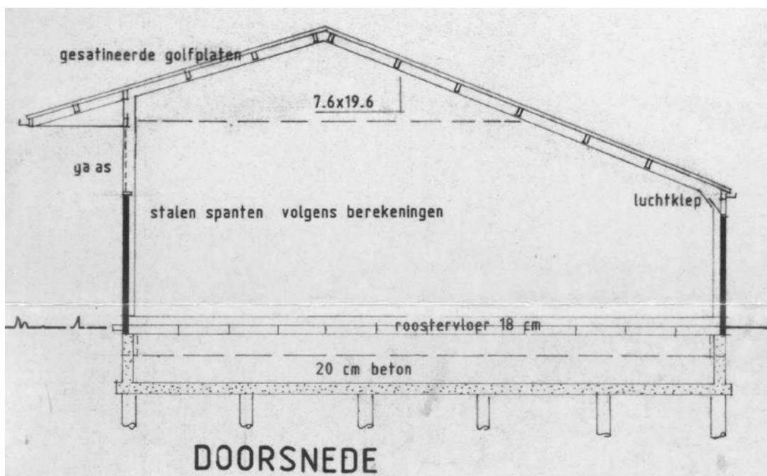
Afbeelding 7: Doorsnede stalwoningen
