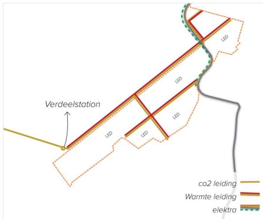
Figuur 7: Verdeling CO 2 en warmteleidingen door het kernglastuinbouwgebied.
