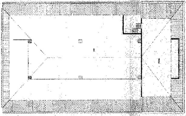
- PLATTEGROND VERDERIJ -
