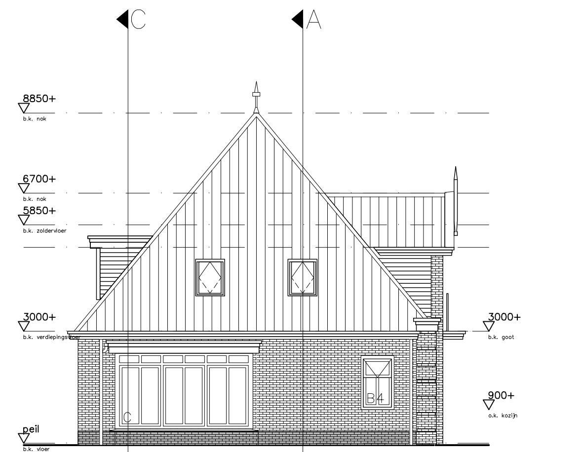
linkerzijgevel BO-1 versie 01/12/2010
