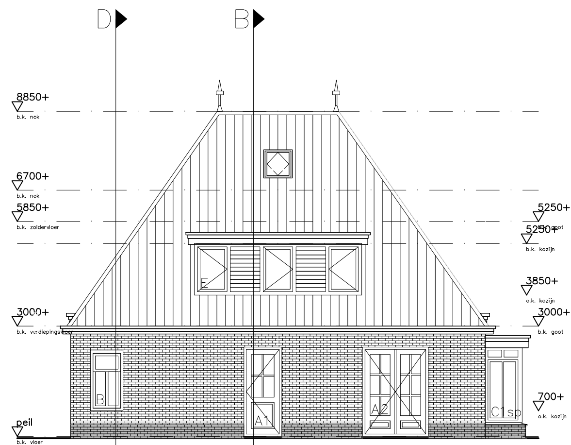
achtergevel BO-1 versie 01/12/2010
