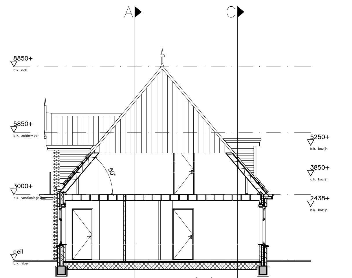
doorsnede D-D BO-1 versie 01/12/2010
