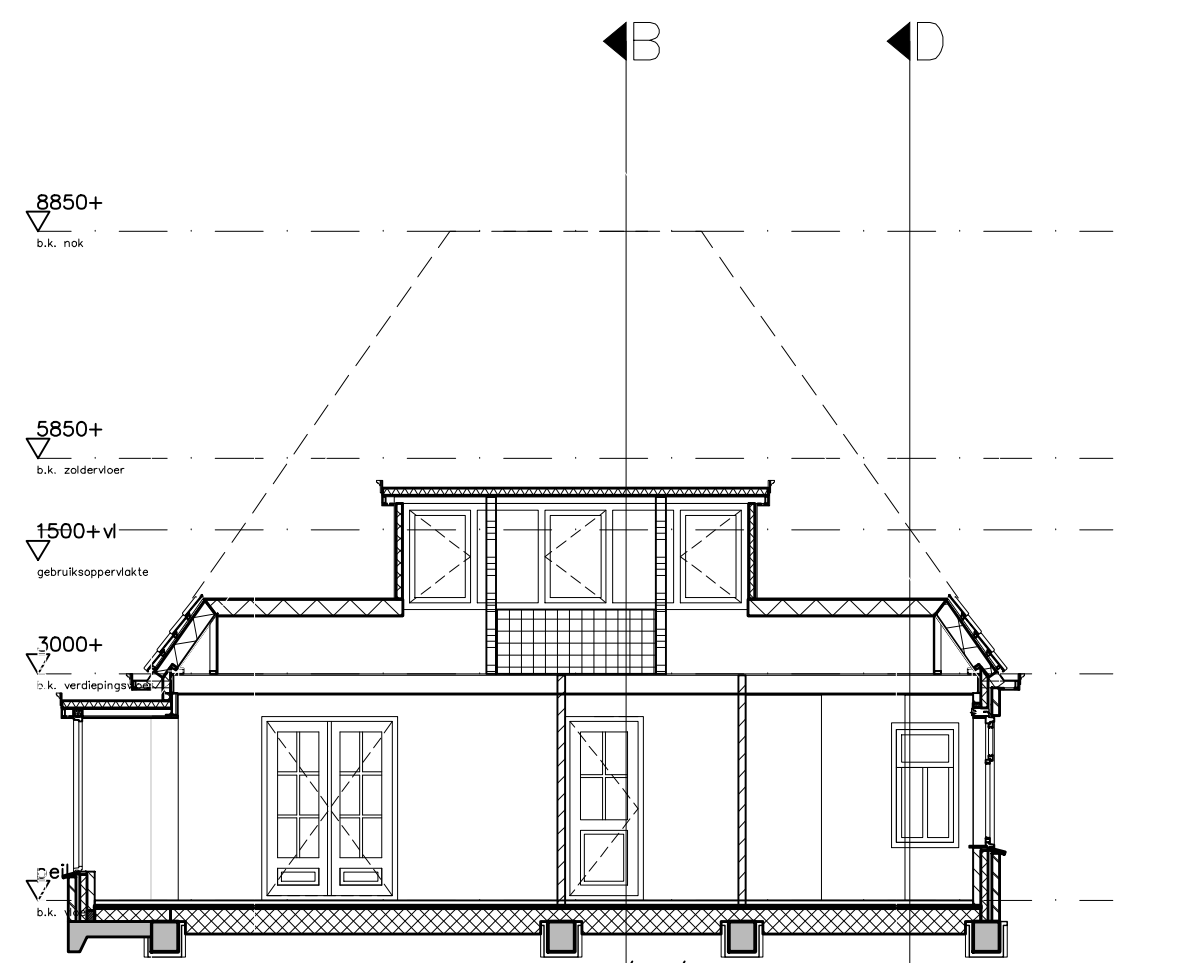
doorsnede C-C BO-1 versie 01/12/2010
