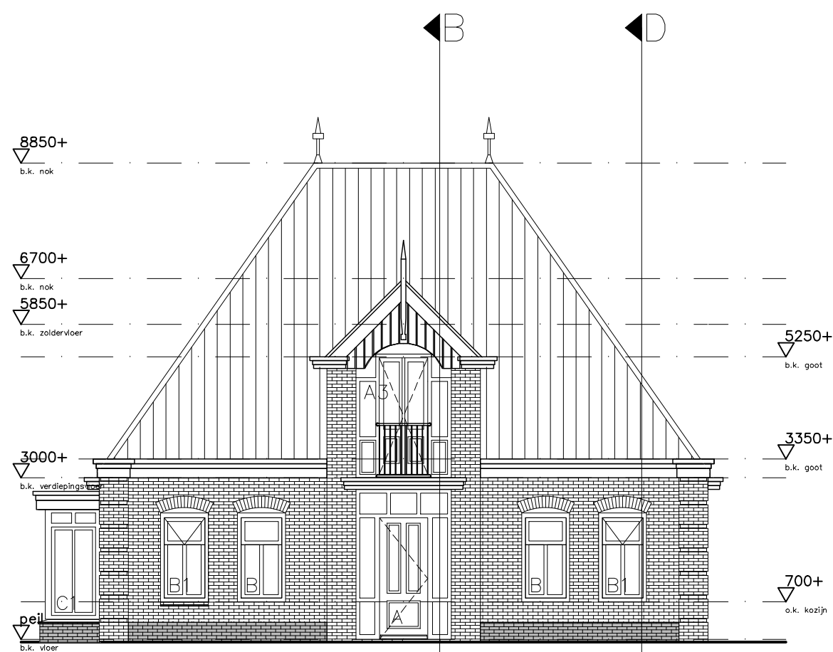
voorgevel BO-1 versie 01/12/2010
