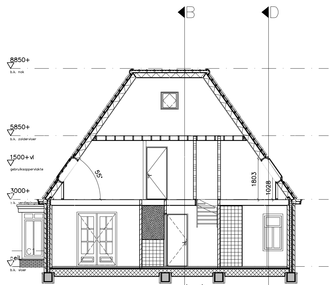
doorsnede A-A BO-1 versie 01/12/2010
