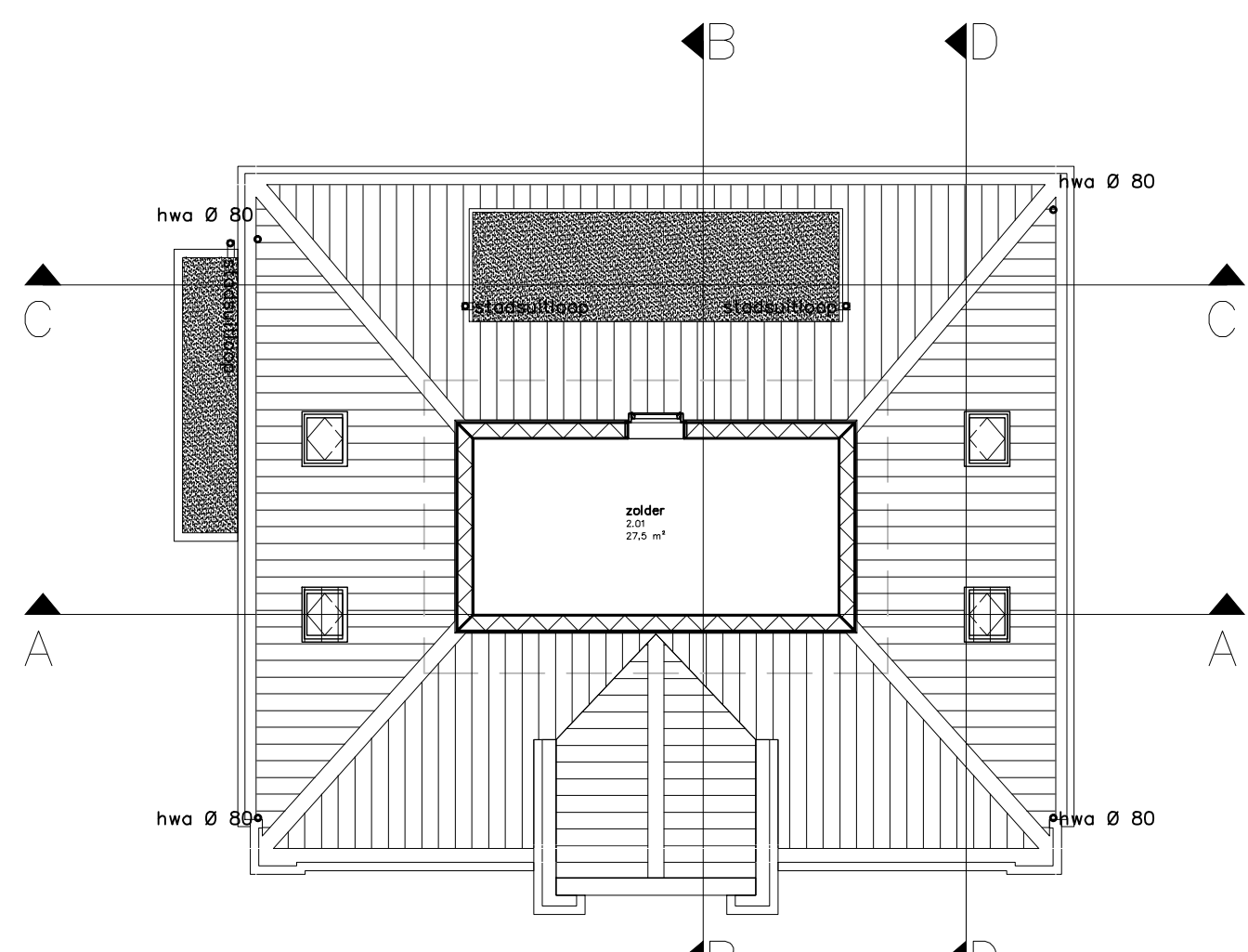
zolder verdieping BO-1 versie 01/12/2010
