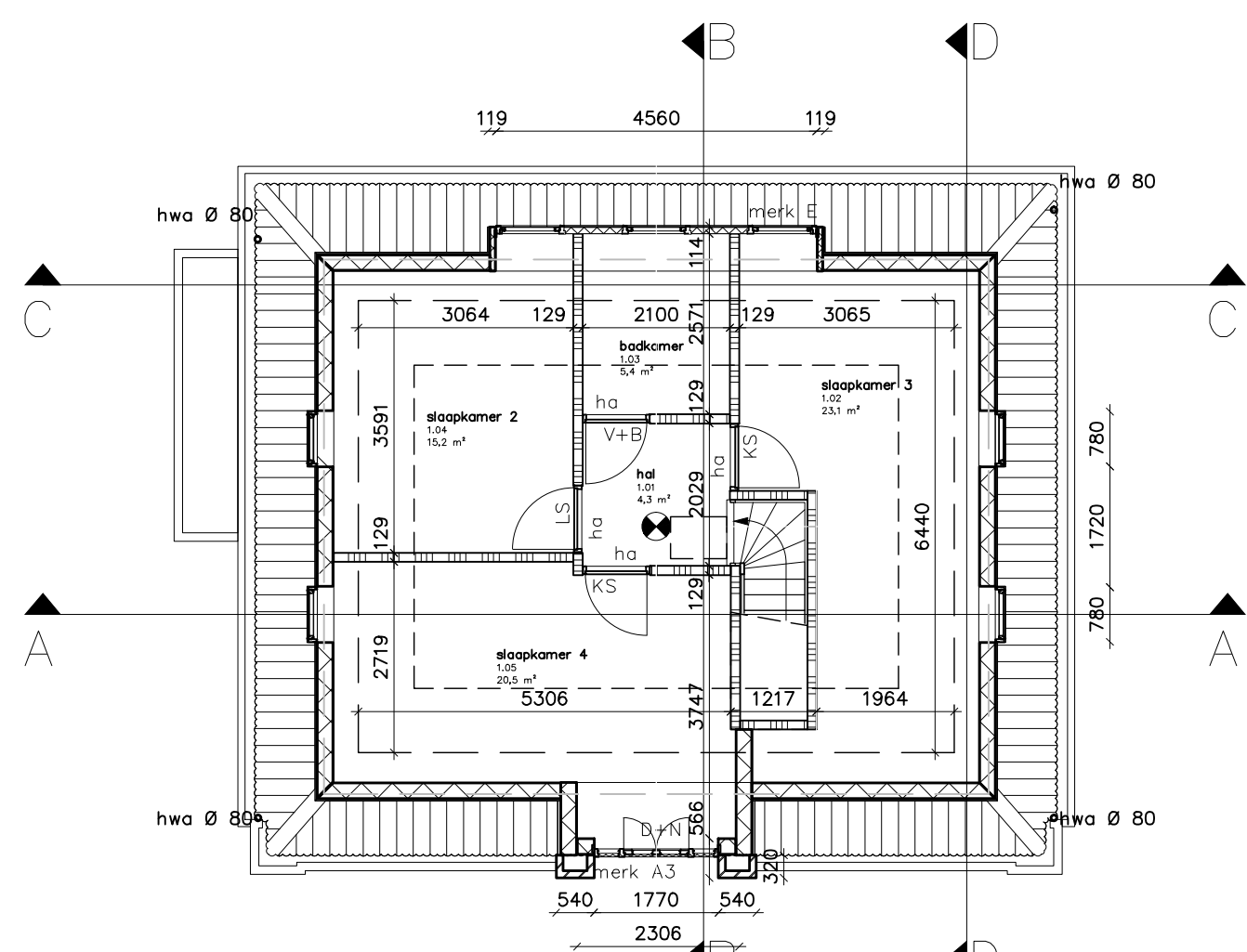
eerste verdieping BO-1 versie 01/12/2010
