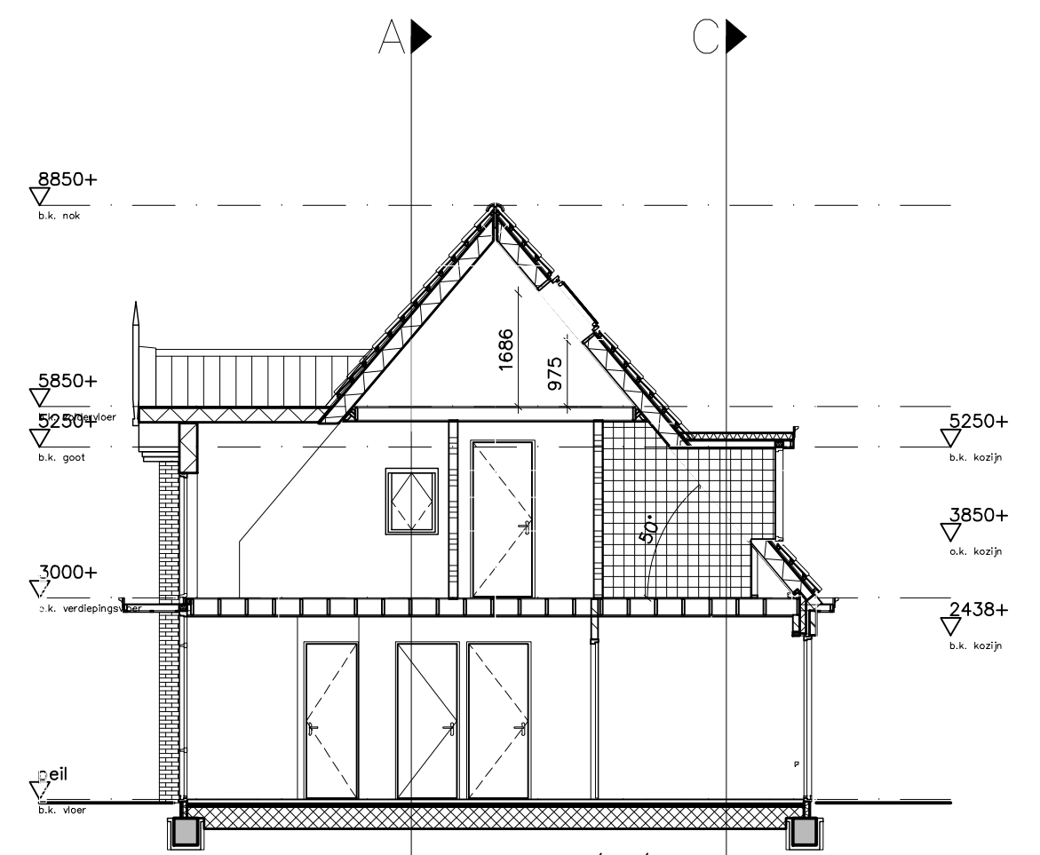
doorsnede B-B BO-1 versie 01/12/2010
