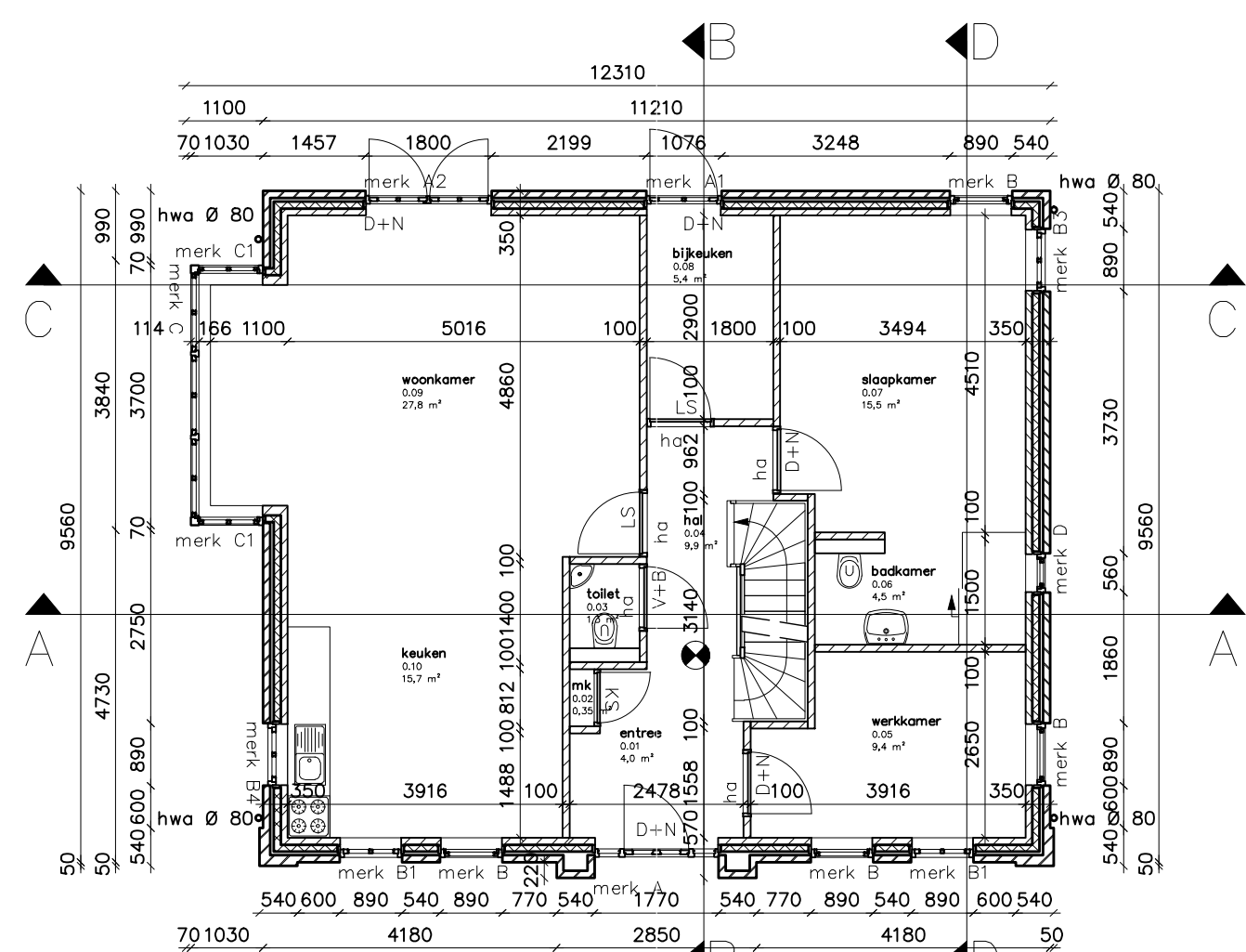
begane grond BO-1 versie 01/12/2010
