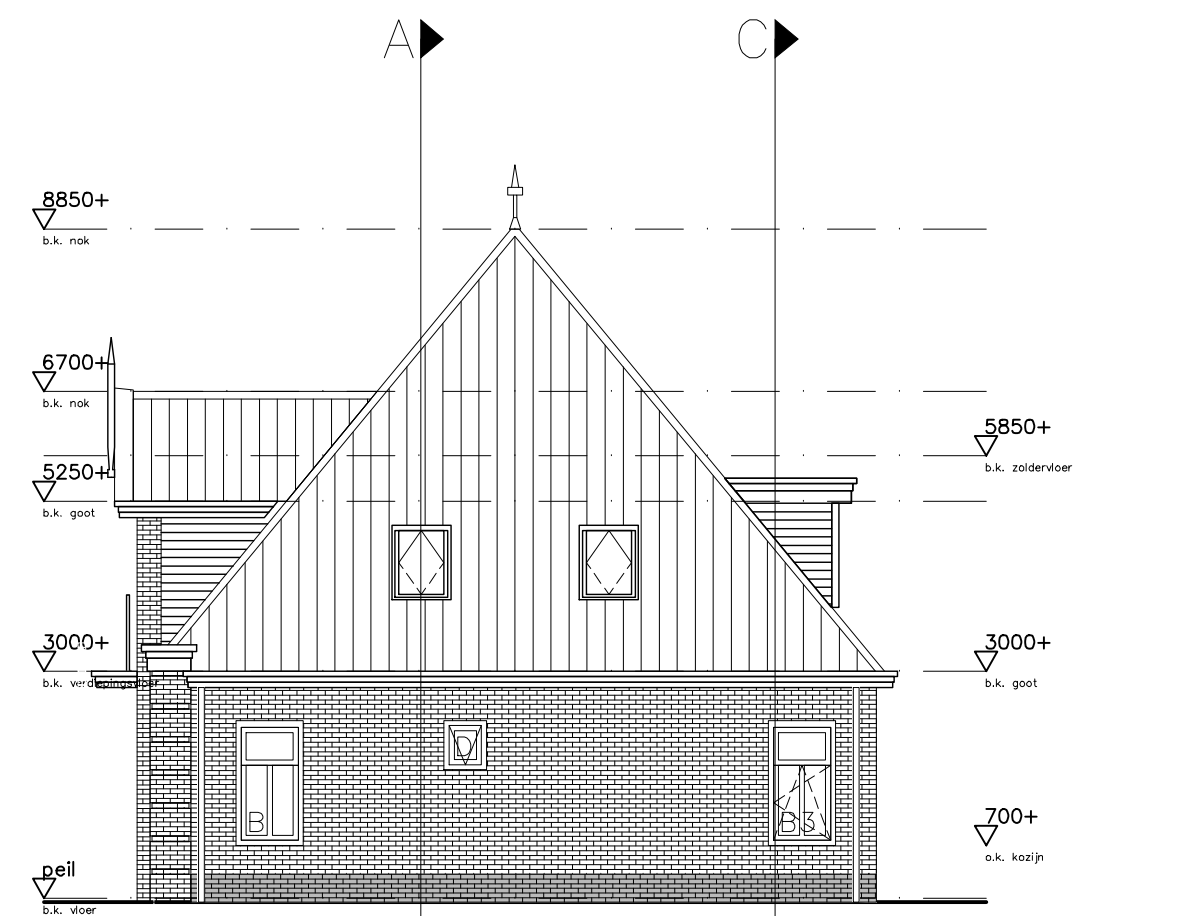
rechterzijgevel BO-1 versie 01/12/2010
