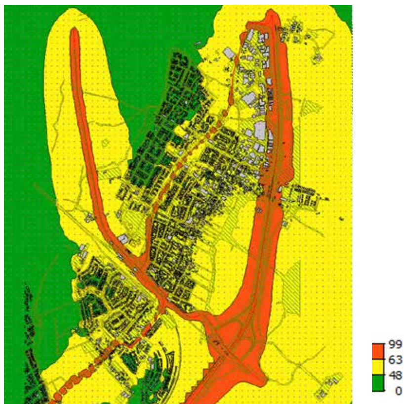
contouren weg- en spoorlawaai (cumulatief)
