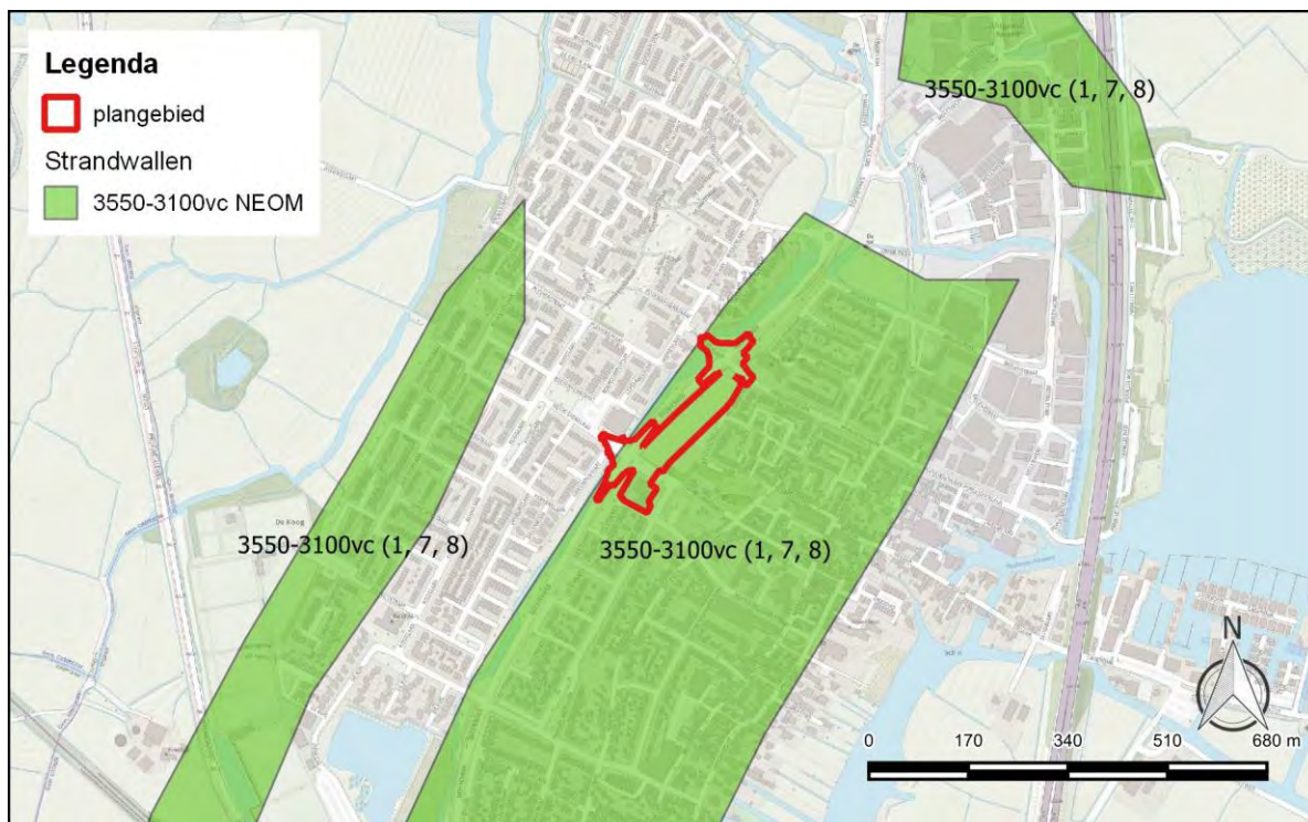
Figuur 7: Ligging van het plangebied op de strandwal die is gevormd tussen 3550 en 3100 voor Chr. (bron: Dalen et al. 2008; Vos et al. 2018; Westerhof et al. 1988).
