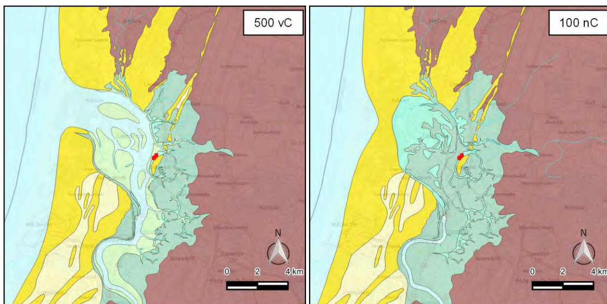
Figuur 4: De landschappelijke situatie in 500 voor Chr. en 100 na Chr. In het plangebied komen duinen voor (geeltinten) en kwelder- en getijdenafzettingen (groentinten). Tussen 500 voor Chr. en 100 na Chr. wordt de monding van het Oer-IJ afgesloten.
