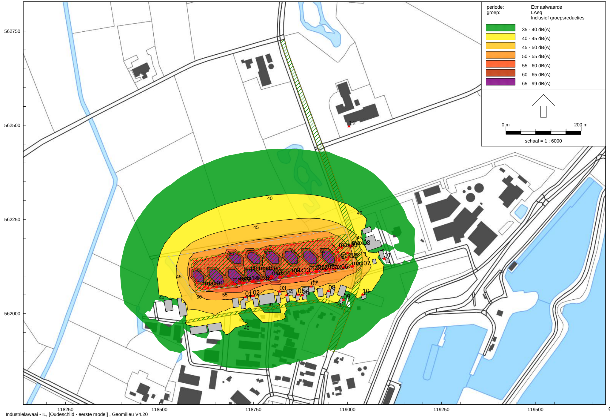
Overzicht van de berekende geluidcontouren
