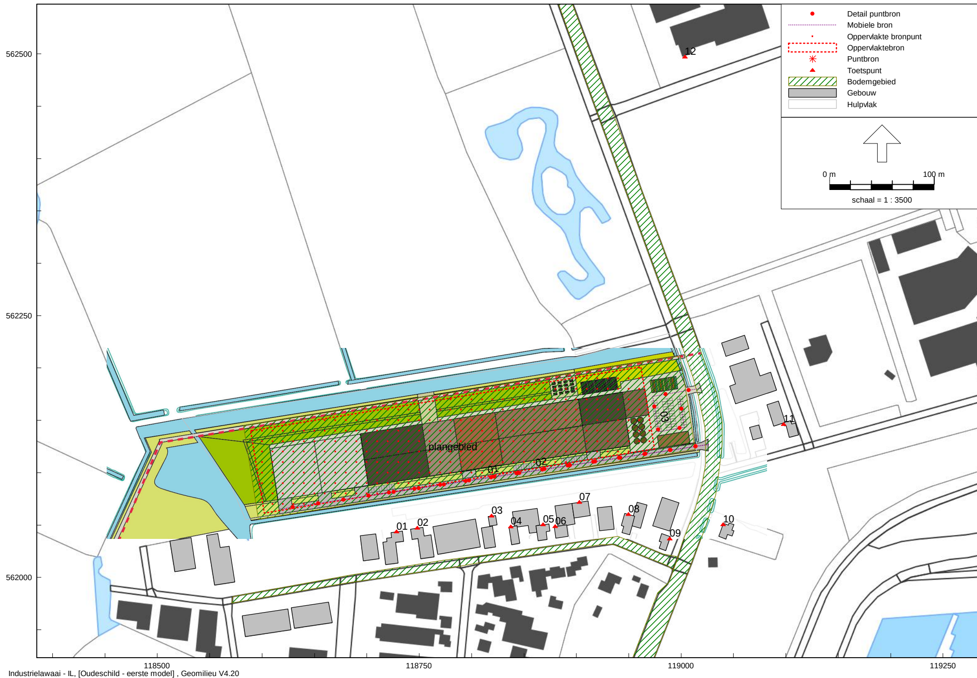
Overzicht rekenmodel met de ligging van de equivalente geluidbronnen
