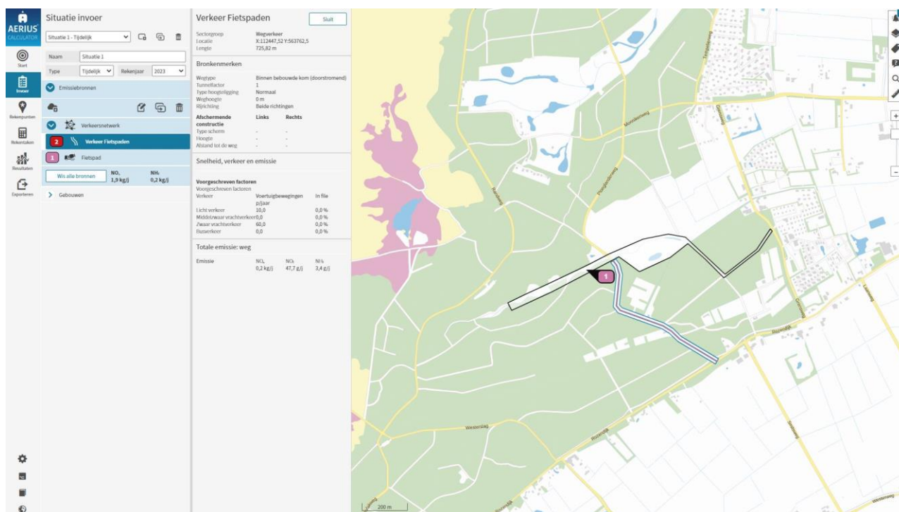
Figuur 18. Invoer tijdelijke situatie, wegverkeer.
