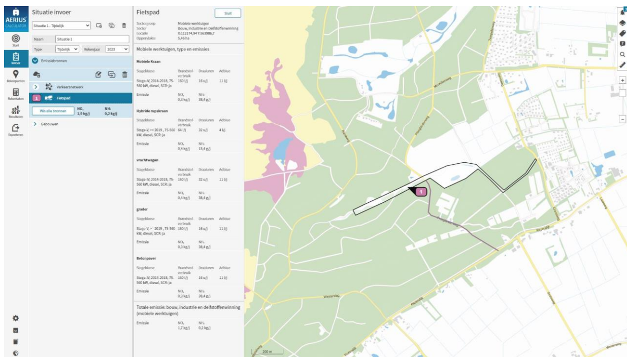
Figuur 17. Invoer tijdelijke situatie, mobiele werktuigen.
